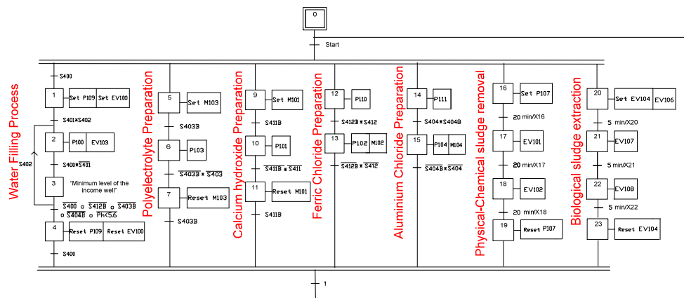
Fig. 7. Level 2 GRAFCET
