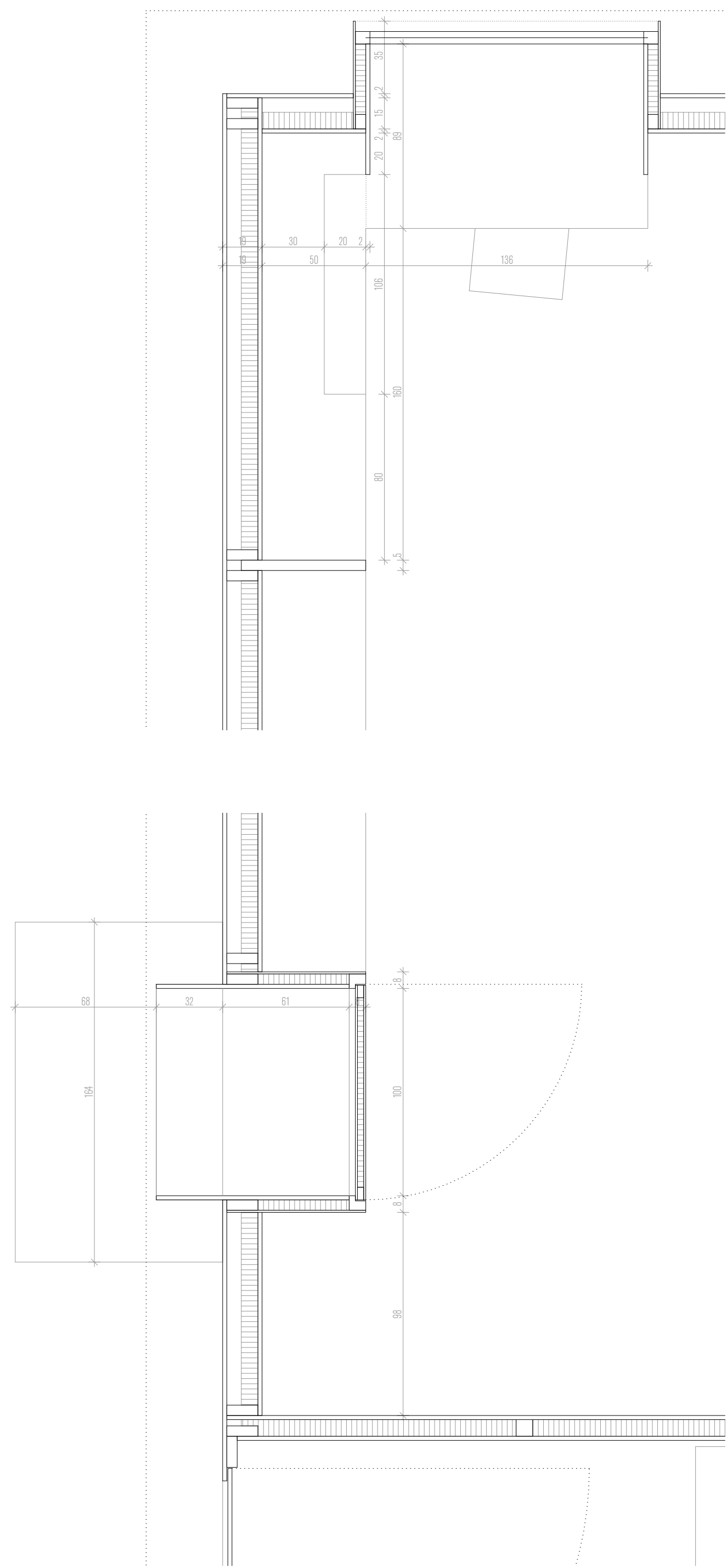
Detall 1:20 del cas 2. Porta d'accés i escriptori-finestra
