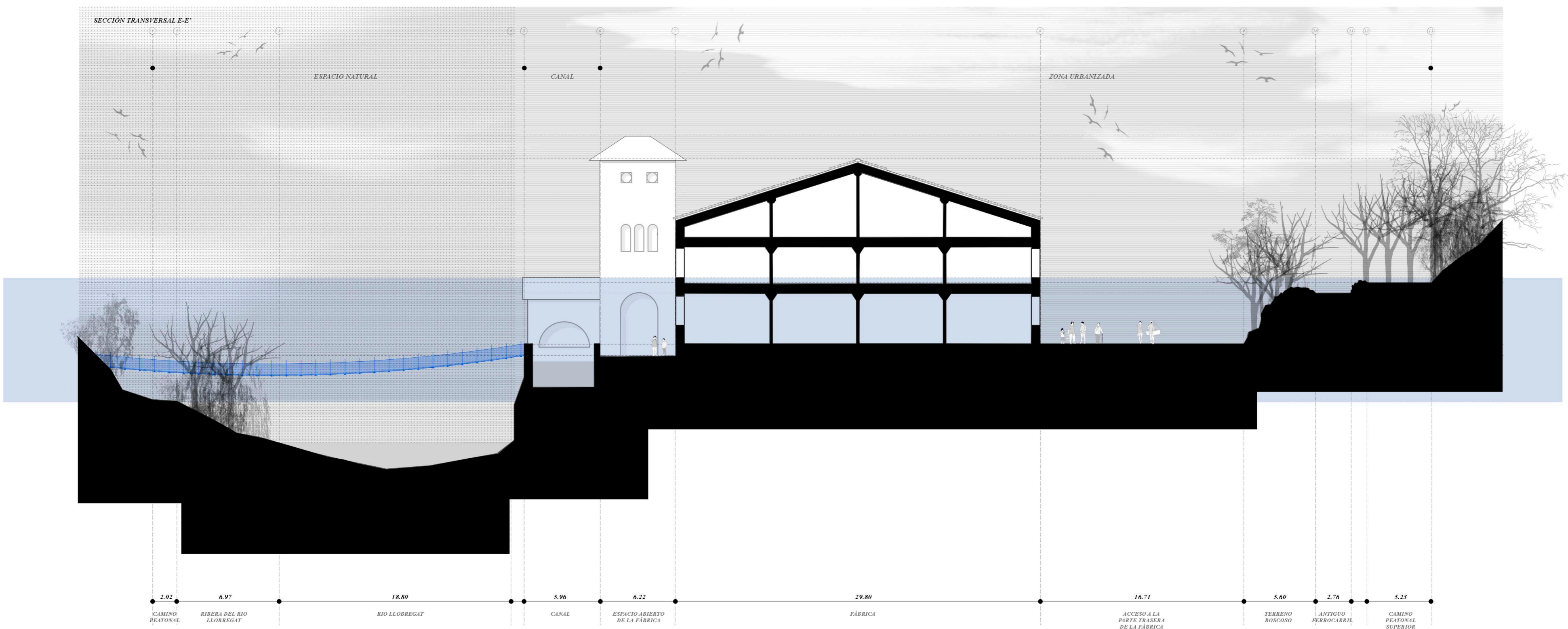
SECCIÓN TRANSVERSAL E-E'
