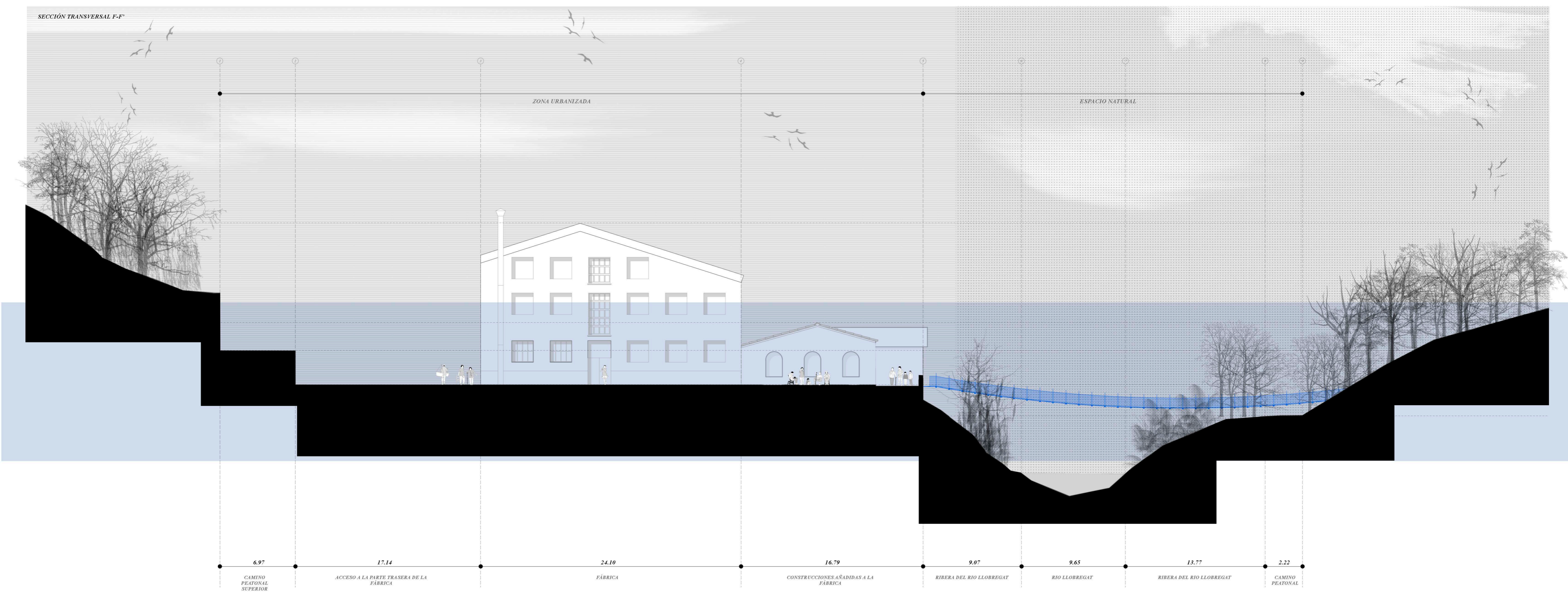
SECCIÓN TRANSVERSAL F-F'
