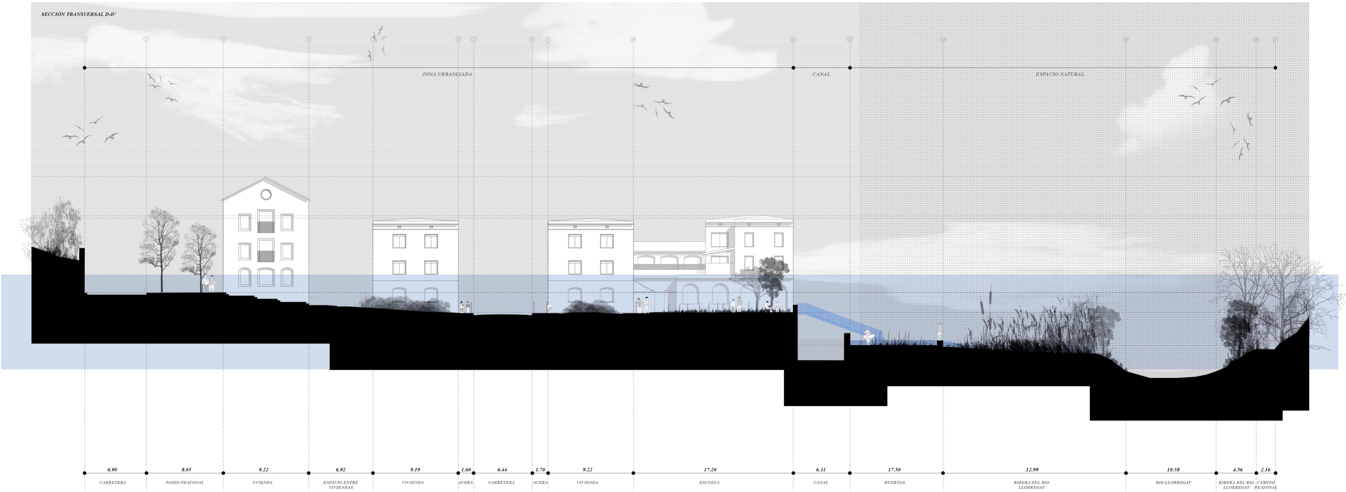
SECCIÓN TRANSVERSAL D-D'
