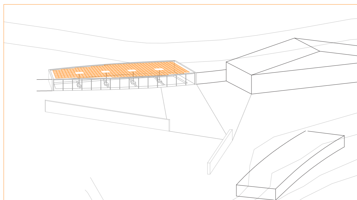
Construcció del forjat reticular amb cassetons recuperables
