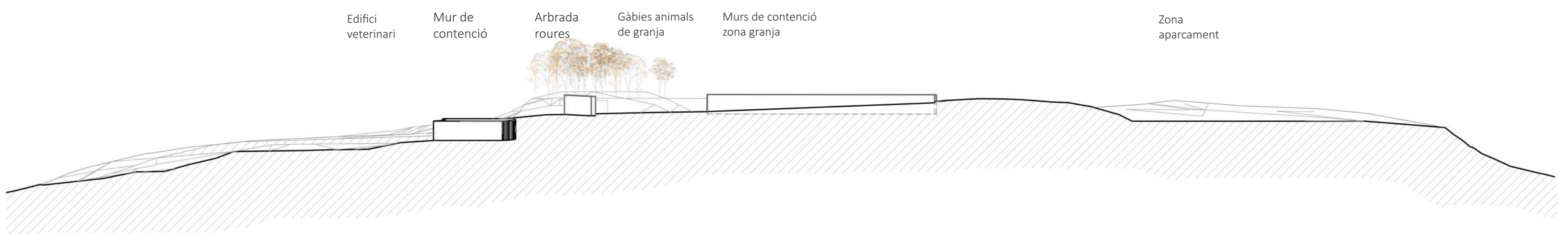
Secció GG'
