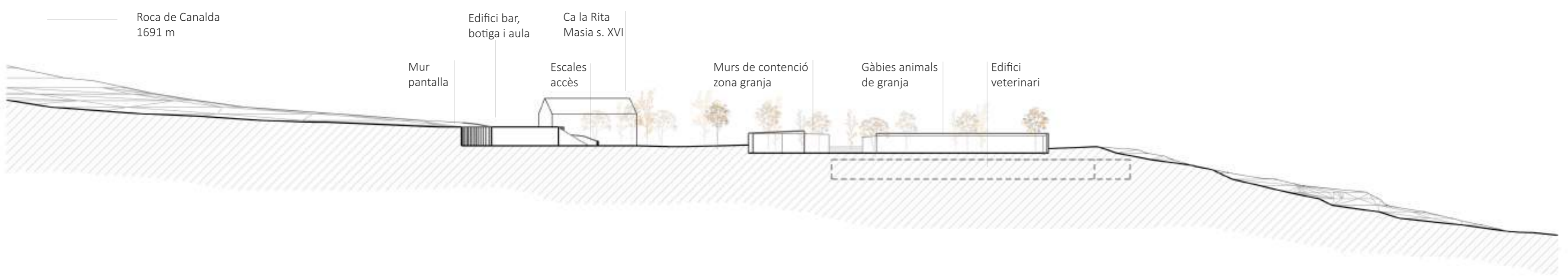
Secció BB'
