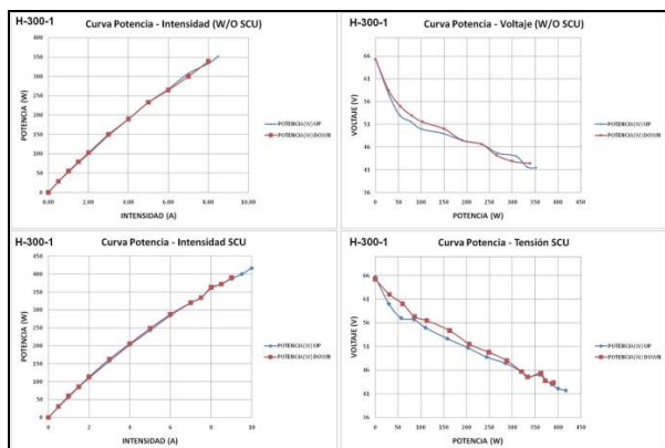
Fig.8: Graficas del ciclo completo (Open Circuit - MaxOutput - Open Circuit) para SCU desactivado y activado.
