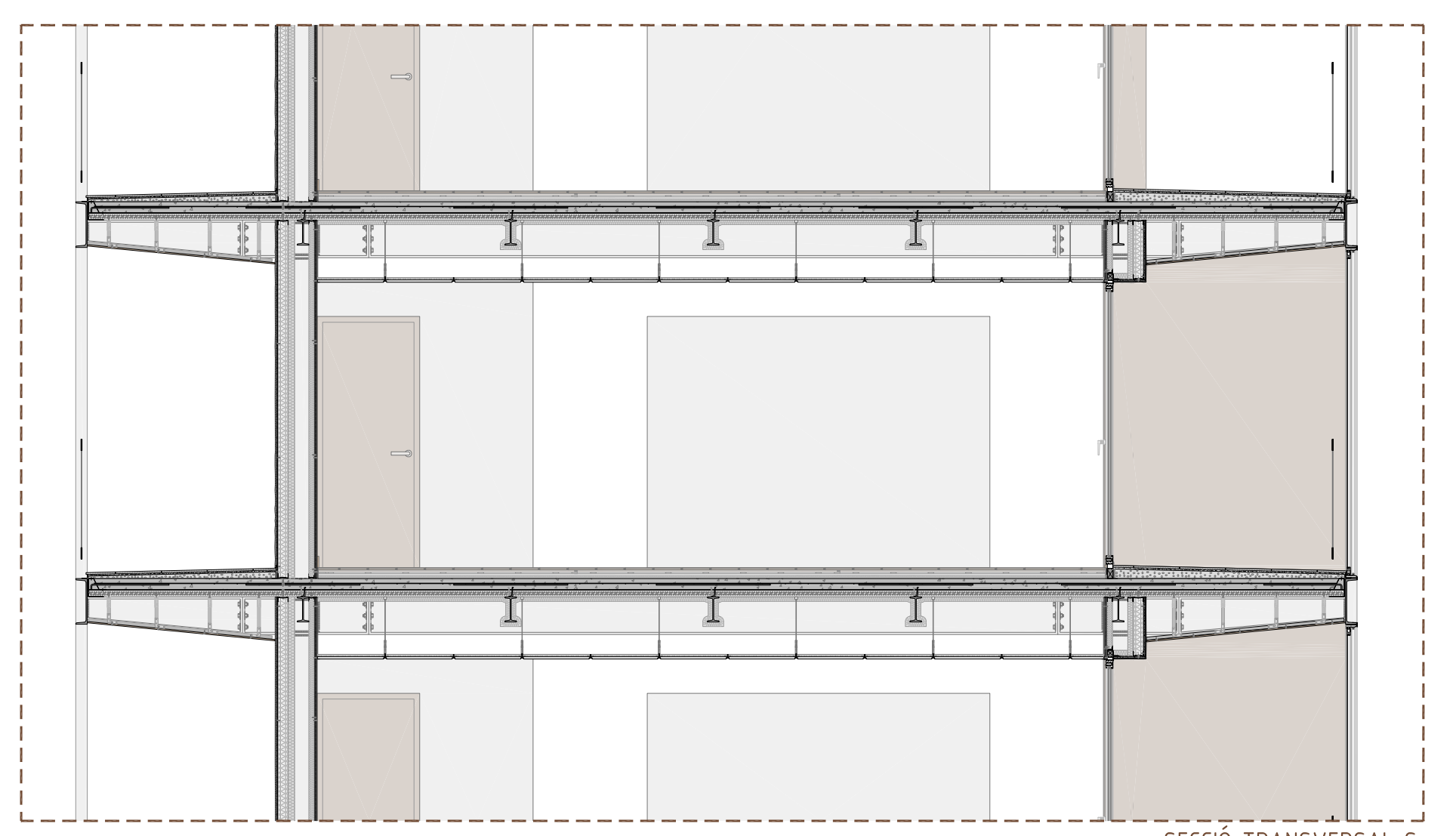
SECCIÓ TRANSVERSAL S2
