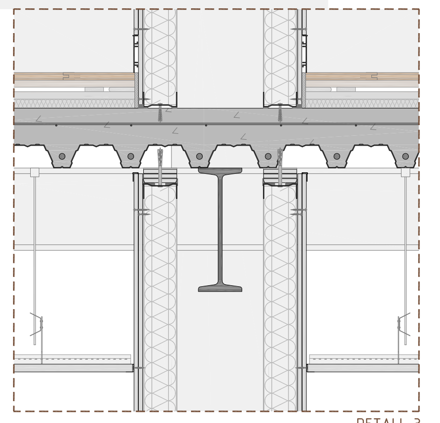
DETALL 3
