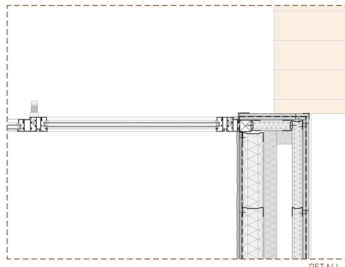
DETALL 1
