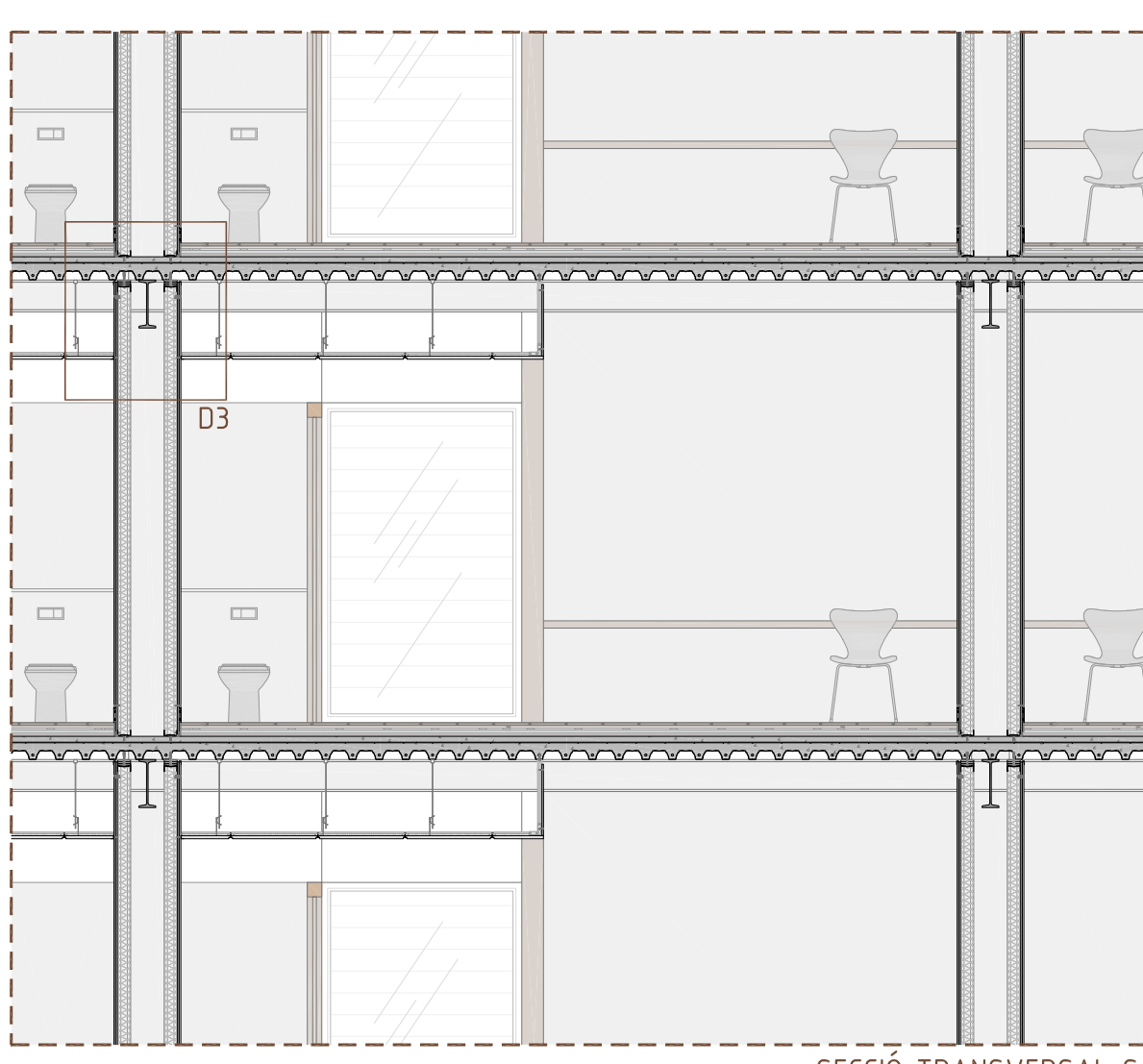
SECCIÓ TRANSVERSAL S1
