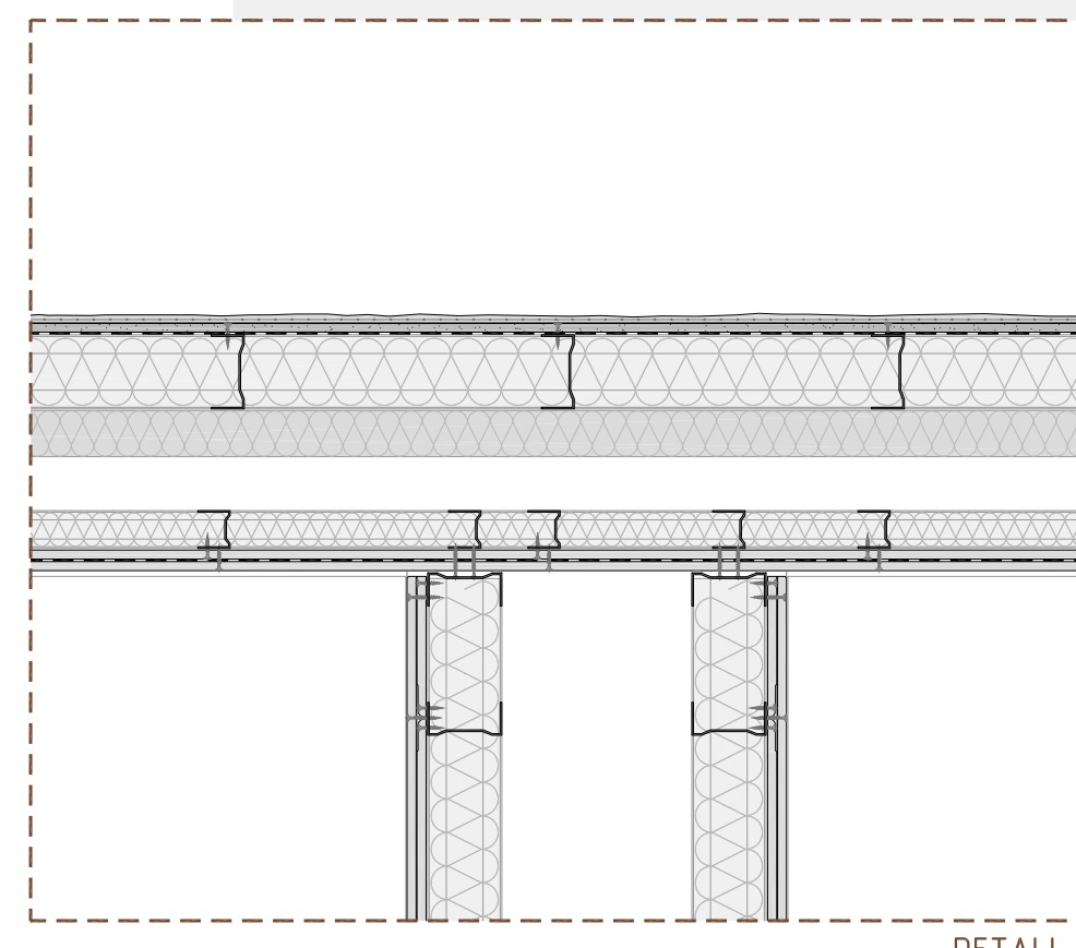
DETALL 2
