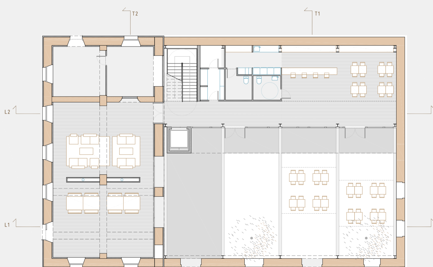
PLANTA BAIXA Nivell 00. +56,5m
