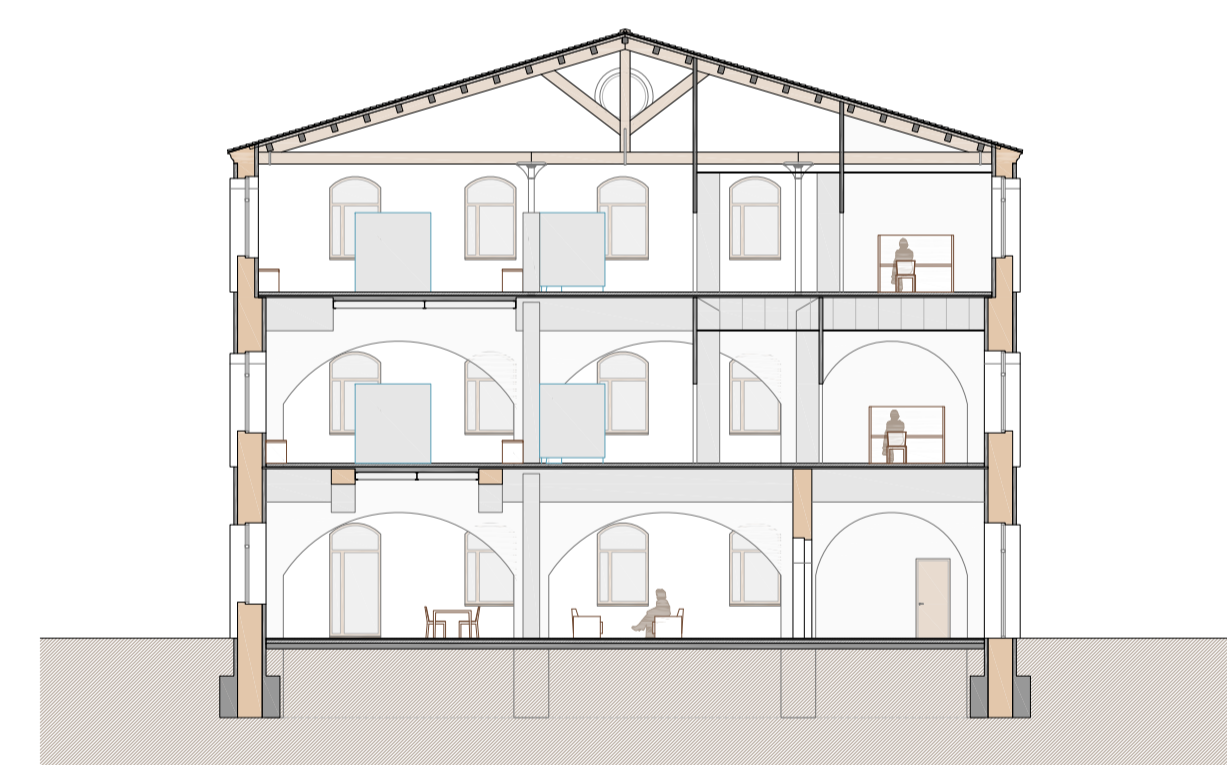
SECCIÓ T2
