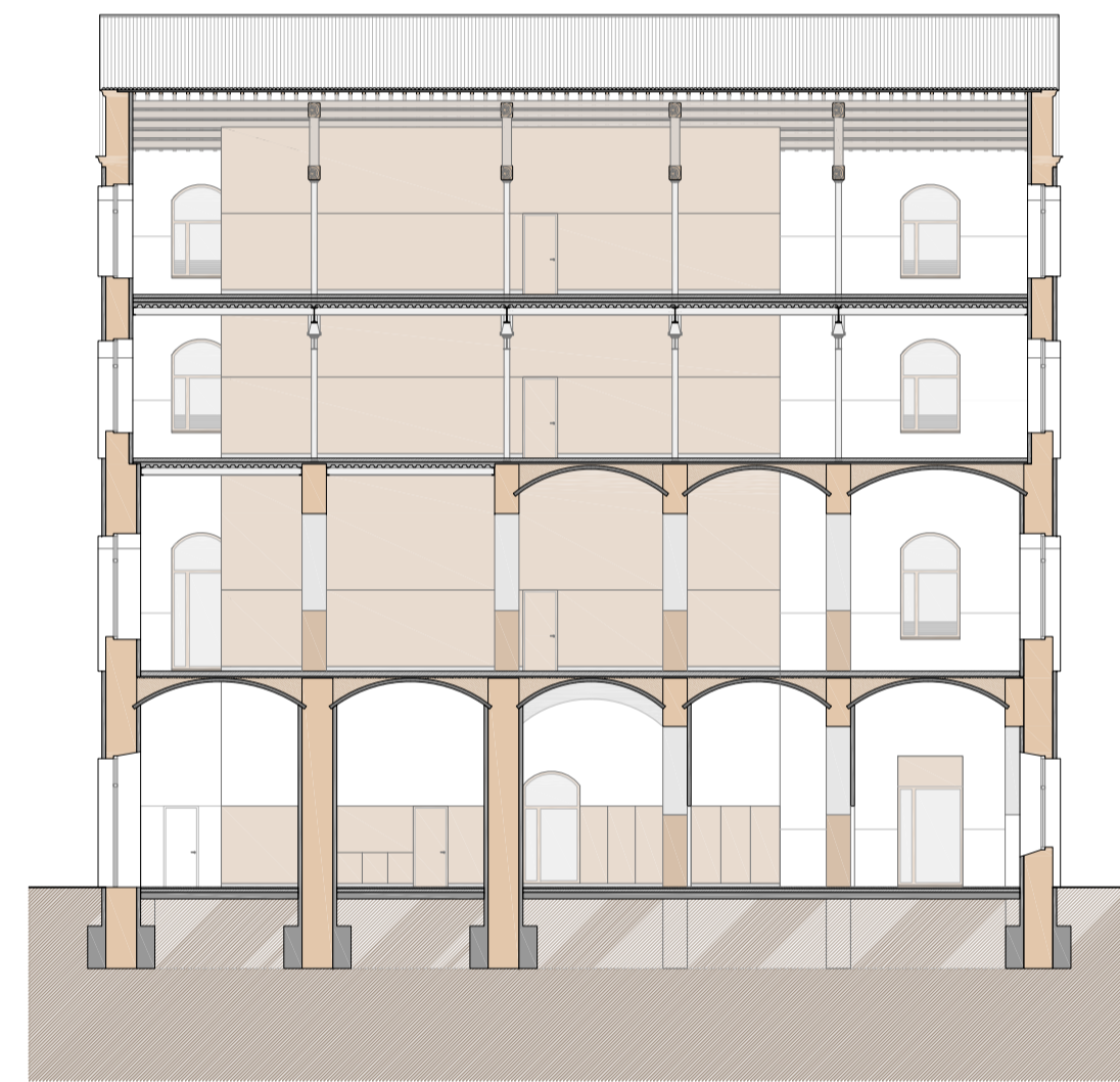
SECCIÓ T1
