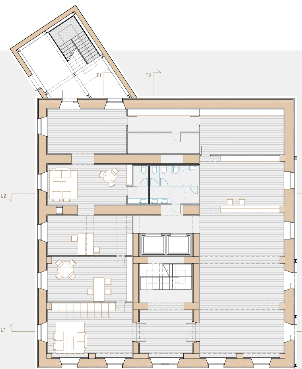
PLANTA BAIXA Nivell 00. +51m
