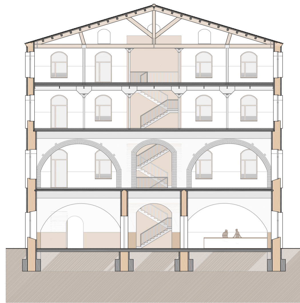
SECCIÓ L1
