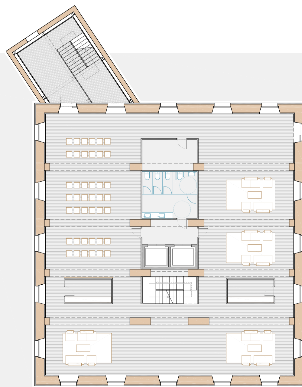
PLANTA PRIMERA Nivell 01. +56,5m
