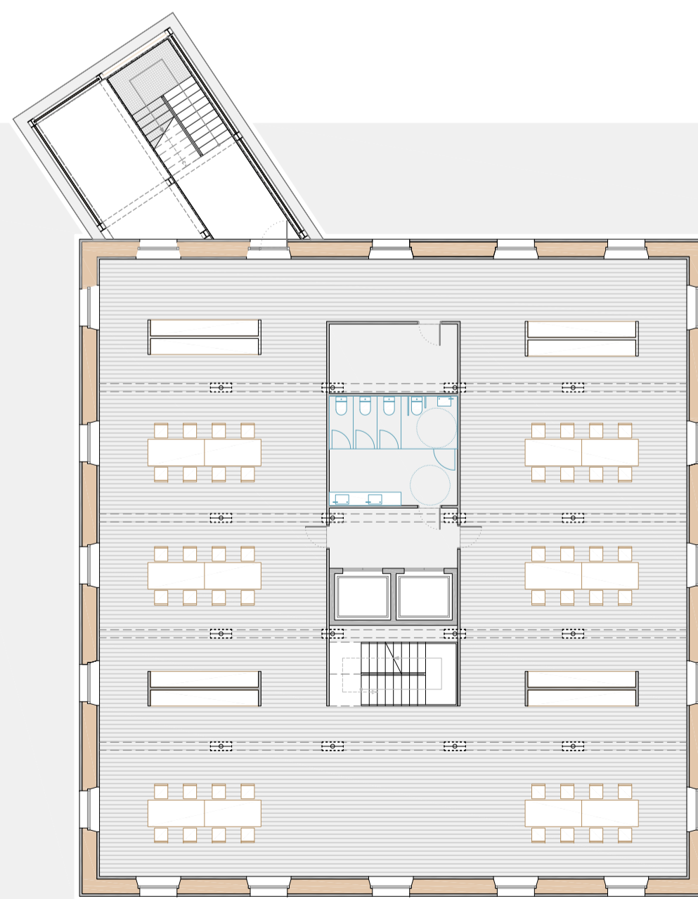
PLANTA SEGONA Nivell 02. +61,5m
