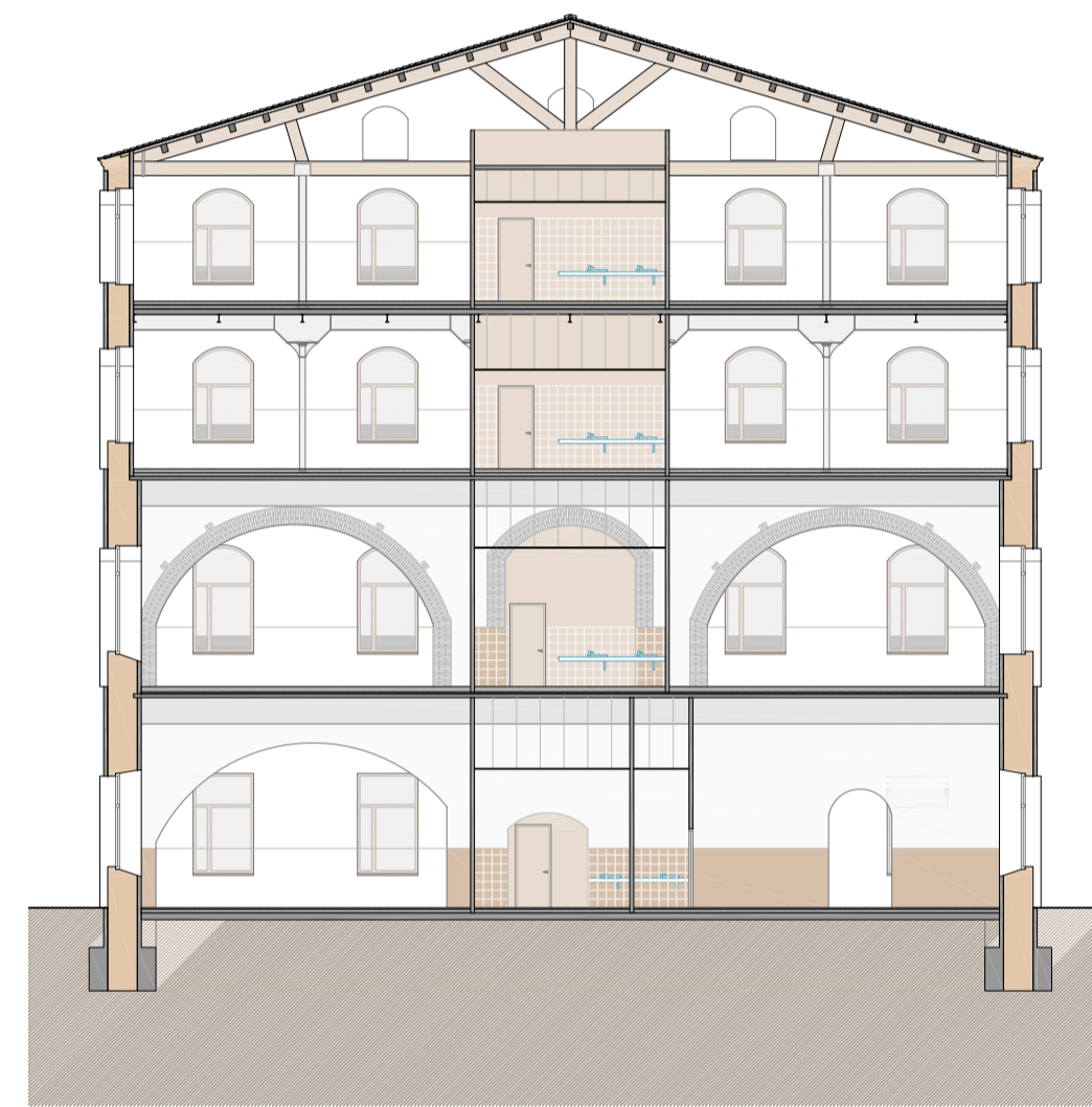
SECCIÓ L2
