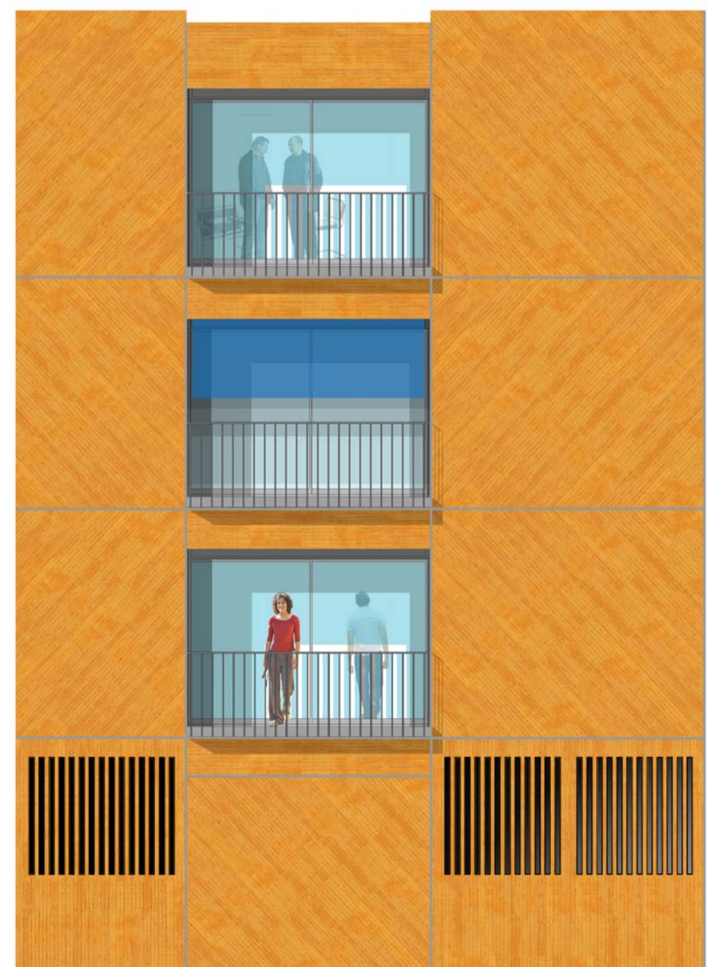
ALÇAT DE MÒDUL DE FAÇANA Materials: Prefabricat formigó. Textures encofrat allistonat / Color: Tenyit òxid ferro. Gelosia ventilació aparcament
