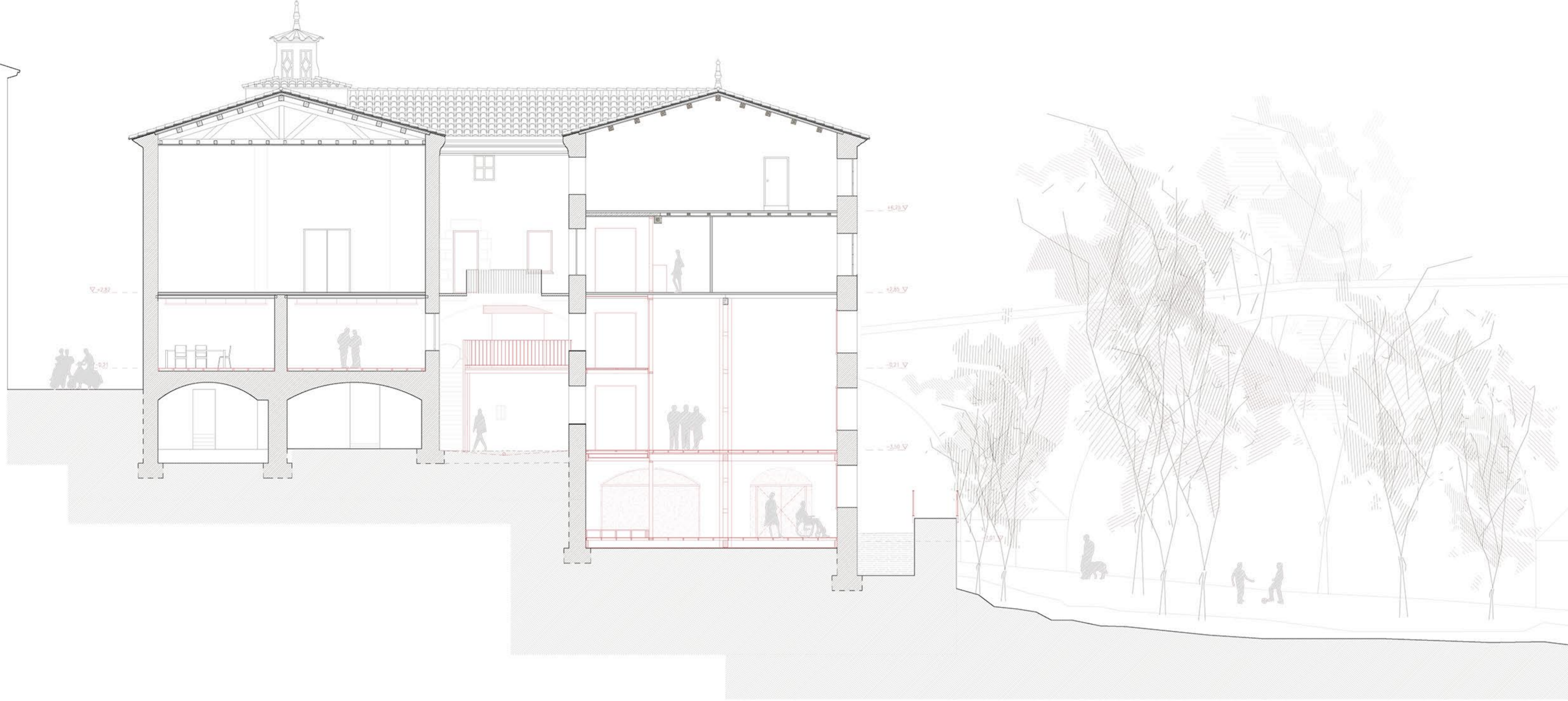
Sección I-I E: 1/100
