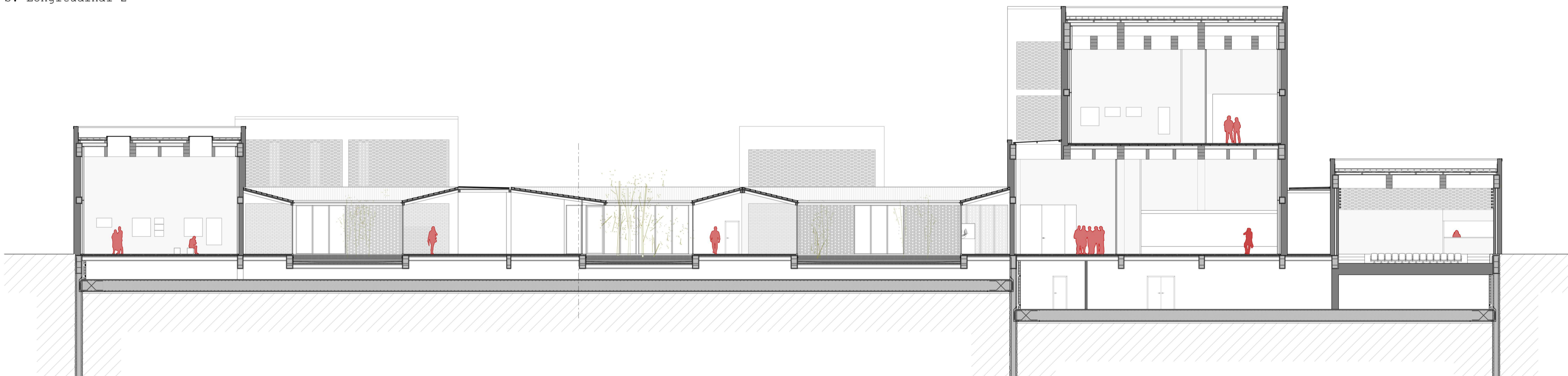
S. Longitudinal 2
