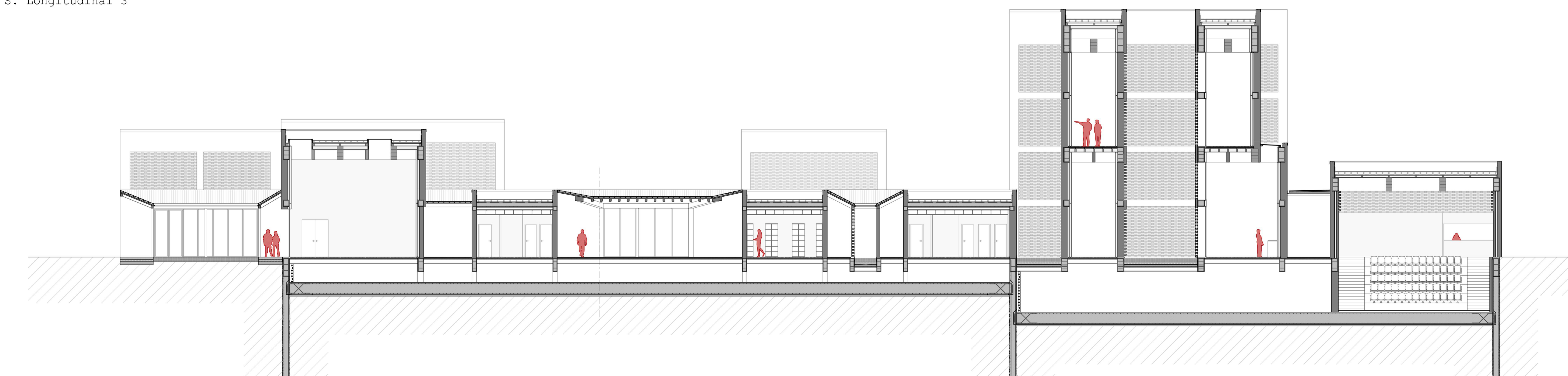
S. Longitudinal 3
