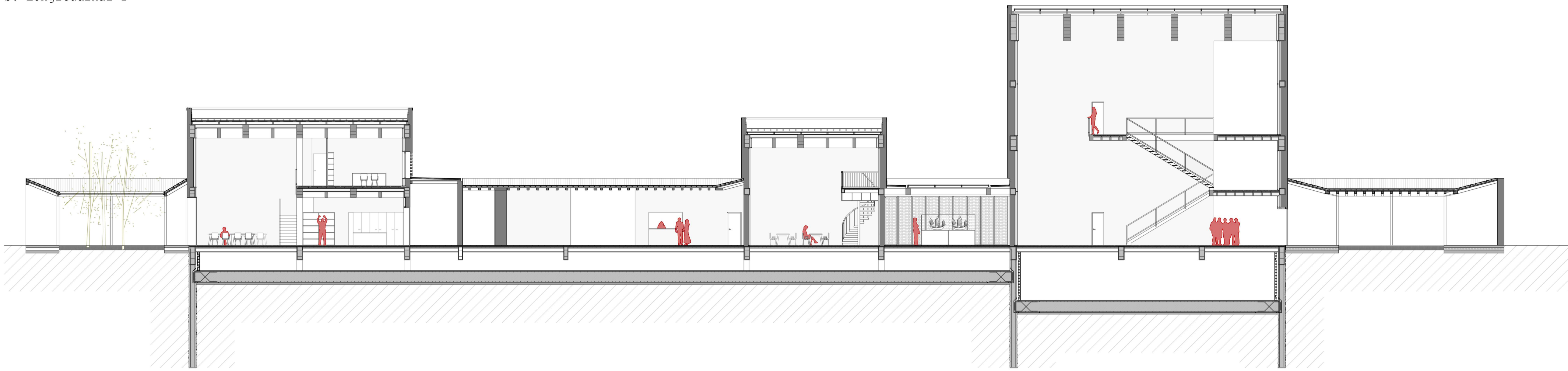
S. Longitudinal 1
