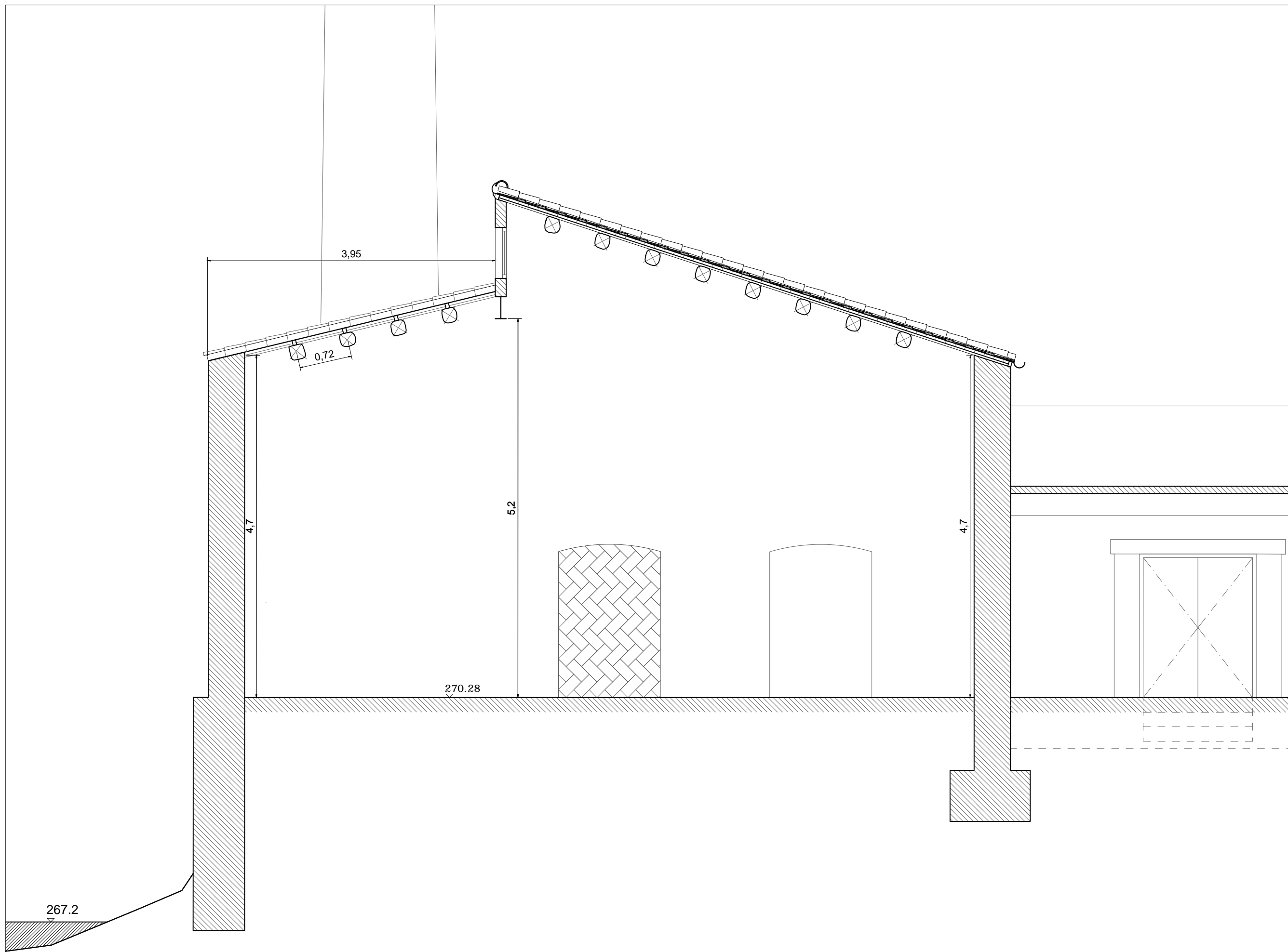
SECCIÓ TRANSVERSAL 2
