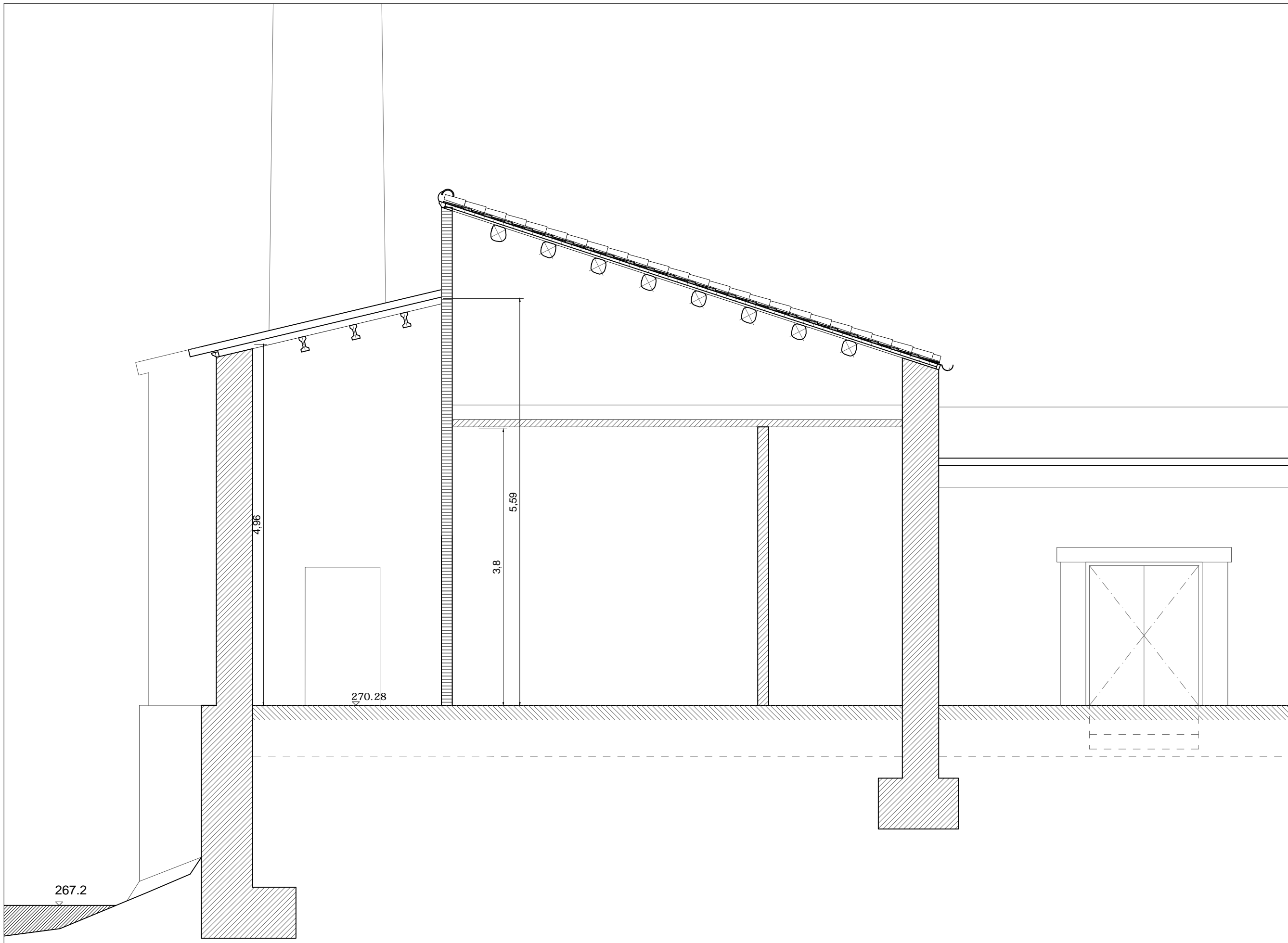
SECCIÓ TRANSVERSAL 1
