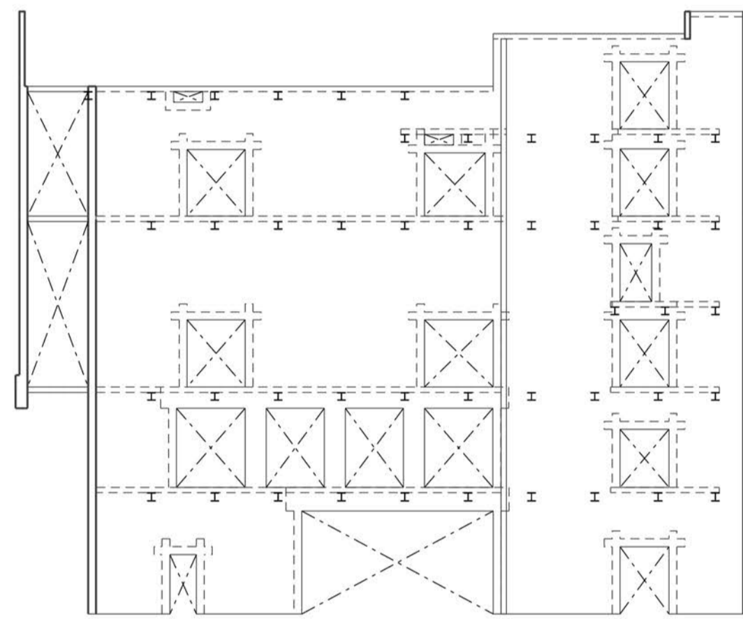
MUR SUD
