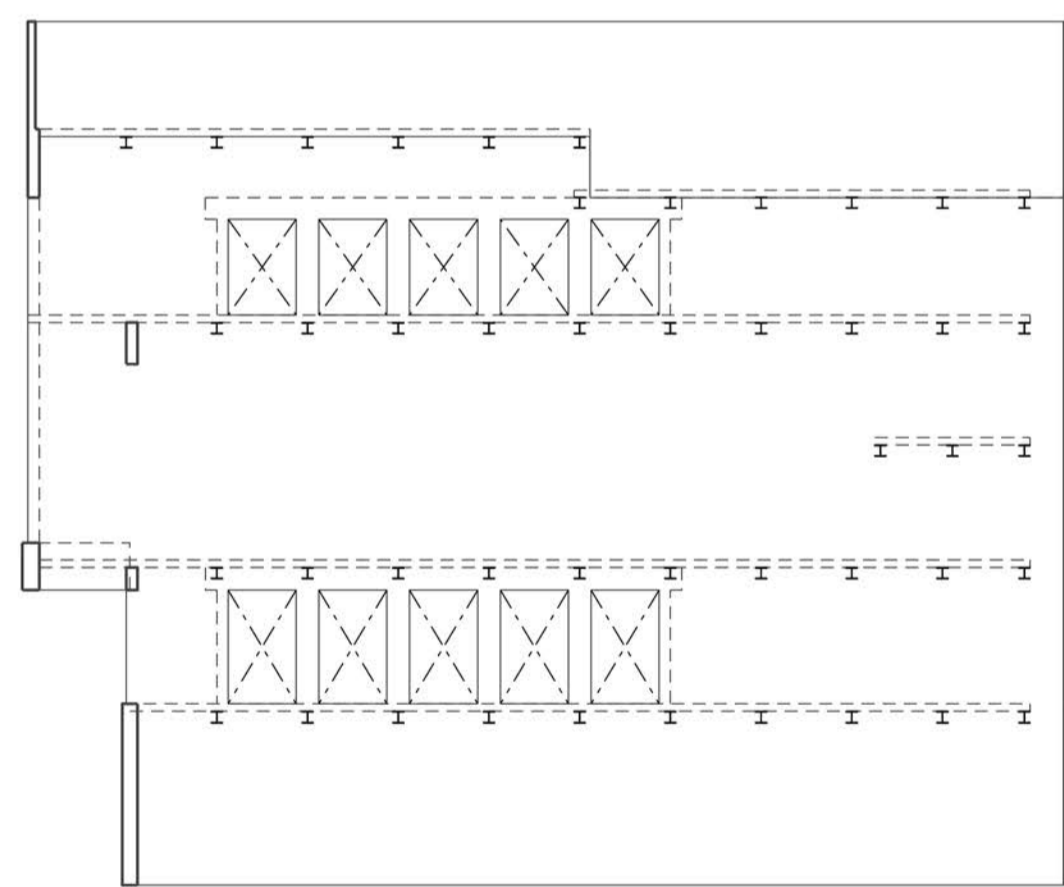
MUR ENTRADA
