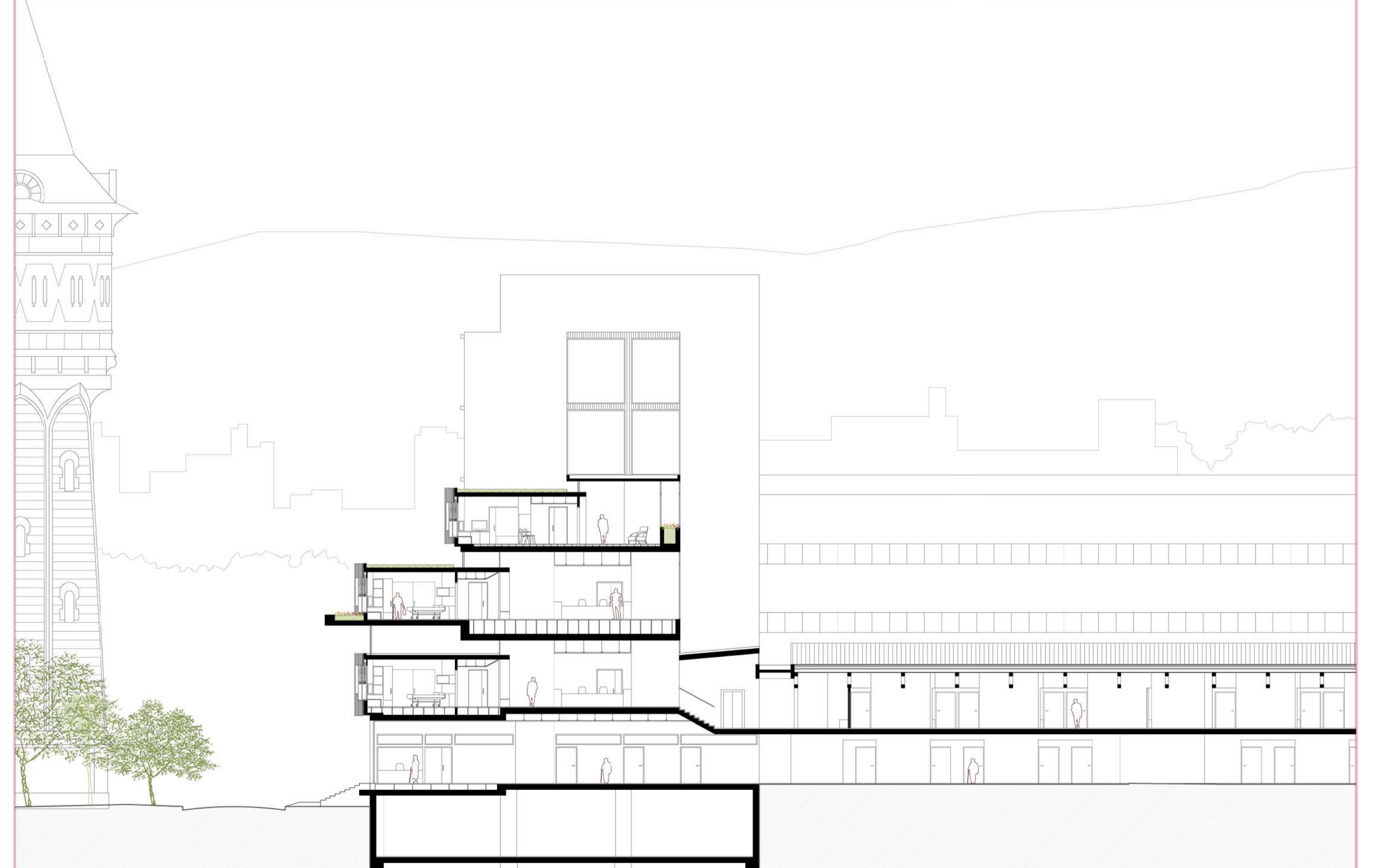
SECCIÓ TRANSVERSAL CC'
