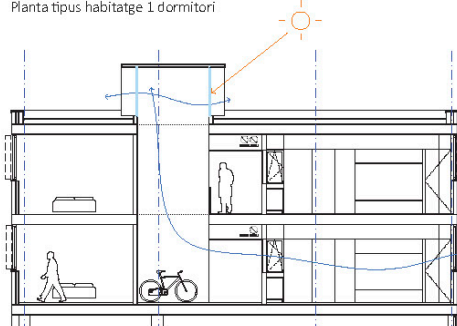
Planta tipus habitatge 1 dormitori
