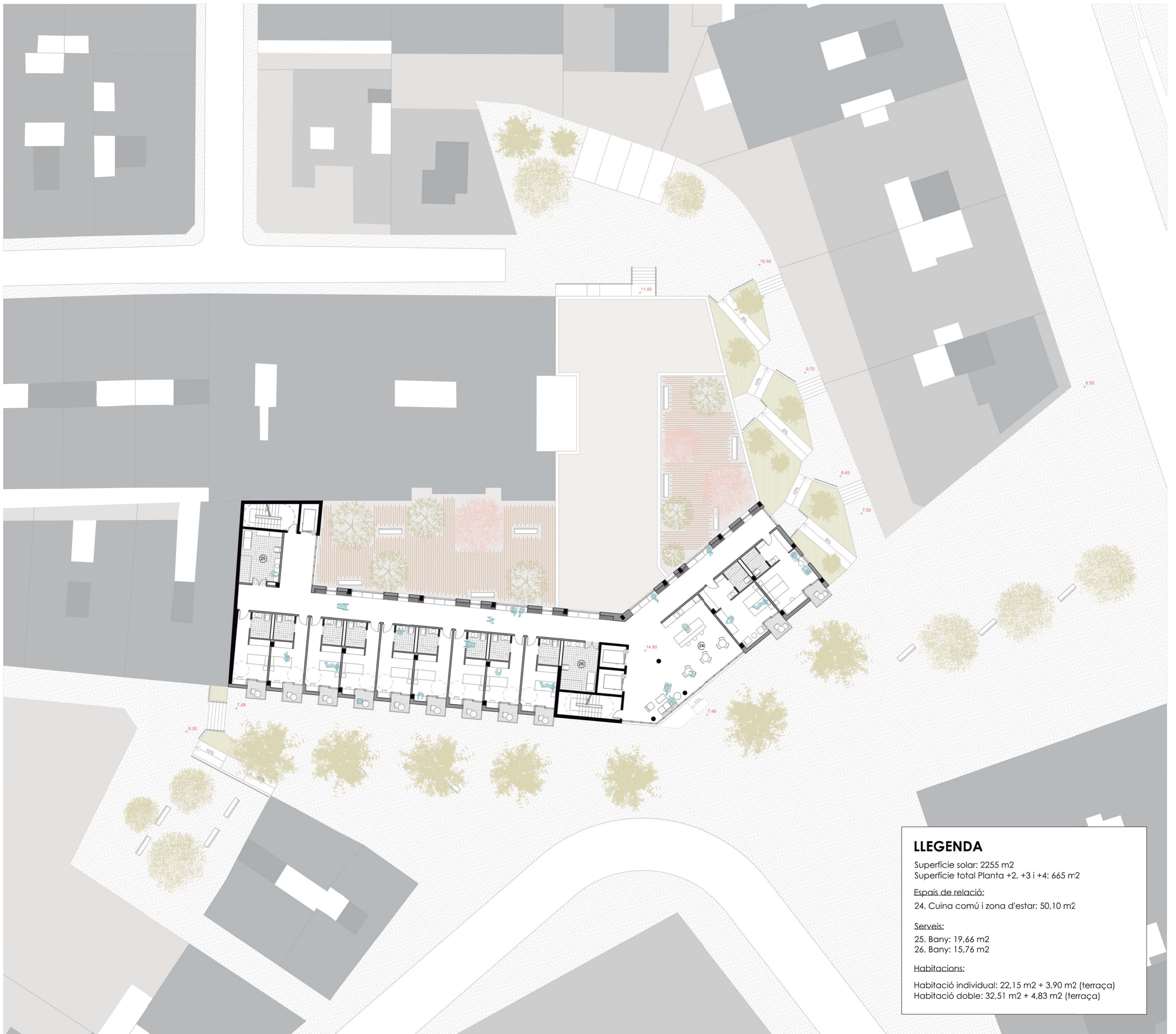
Planta +2 i +3
