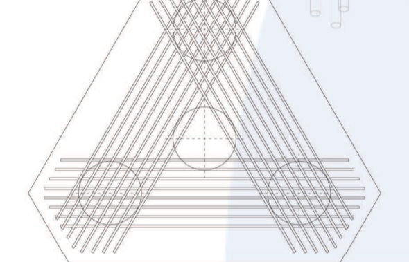
ARMAT INFERIOR DE REFORÇ
