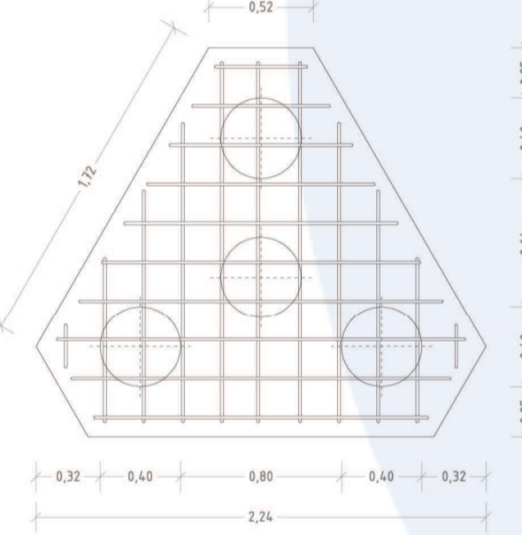
ARMAT INFERIOR DE REFORÇ
