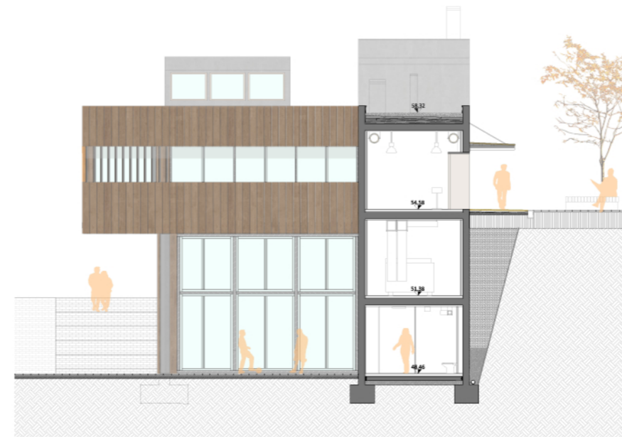
SECCIÓ VERTICAL C-C' FAÇANA NORD
