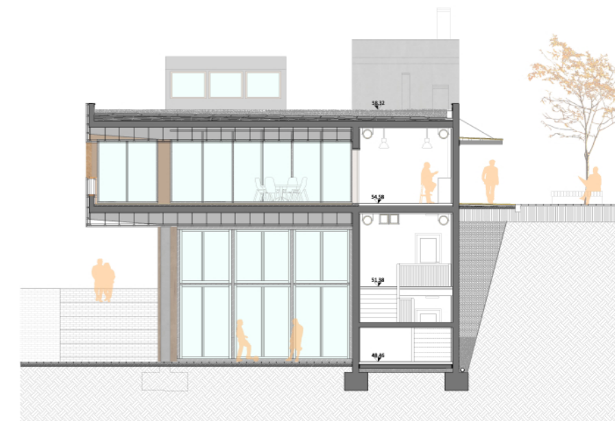
SECCIÓ VERTICAL D-D' FAÇANA NORD
