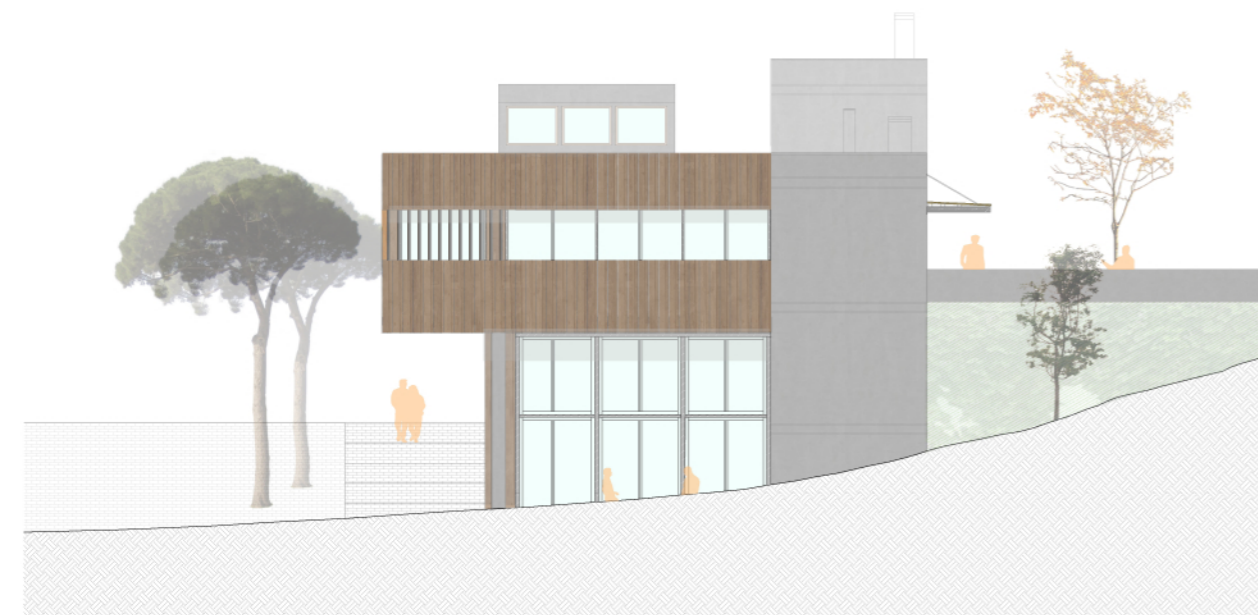
ALÇAT FAÇANA NORD_ sortida directa cap al Museu de la casa ed l'aigua
