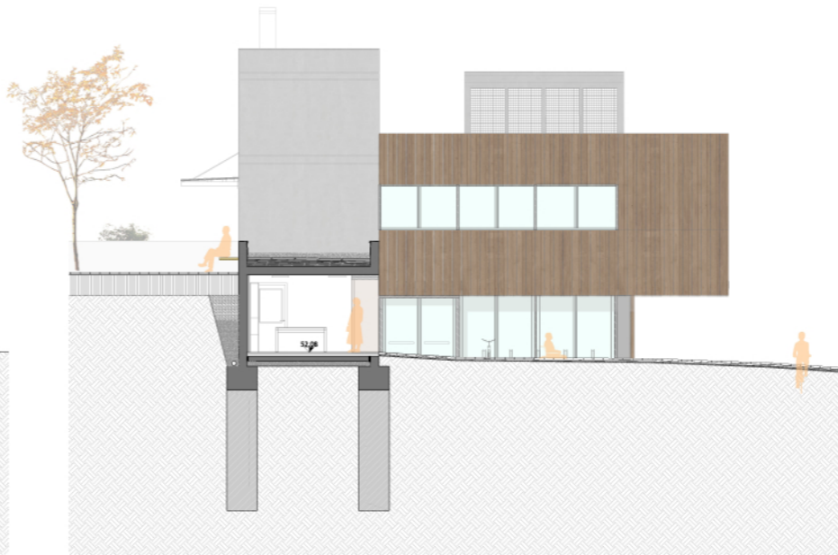
SECCIÓ VERTICAL A-A' FAÇANA SUD
