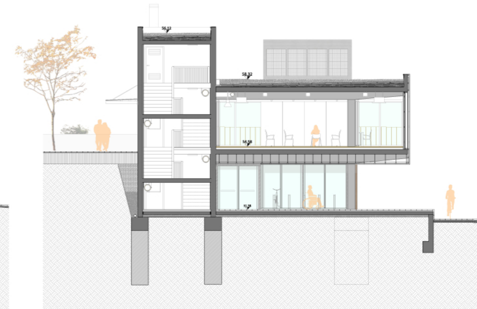
SECCIÓ VERTICAL B-B' FAÇANA SUD
