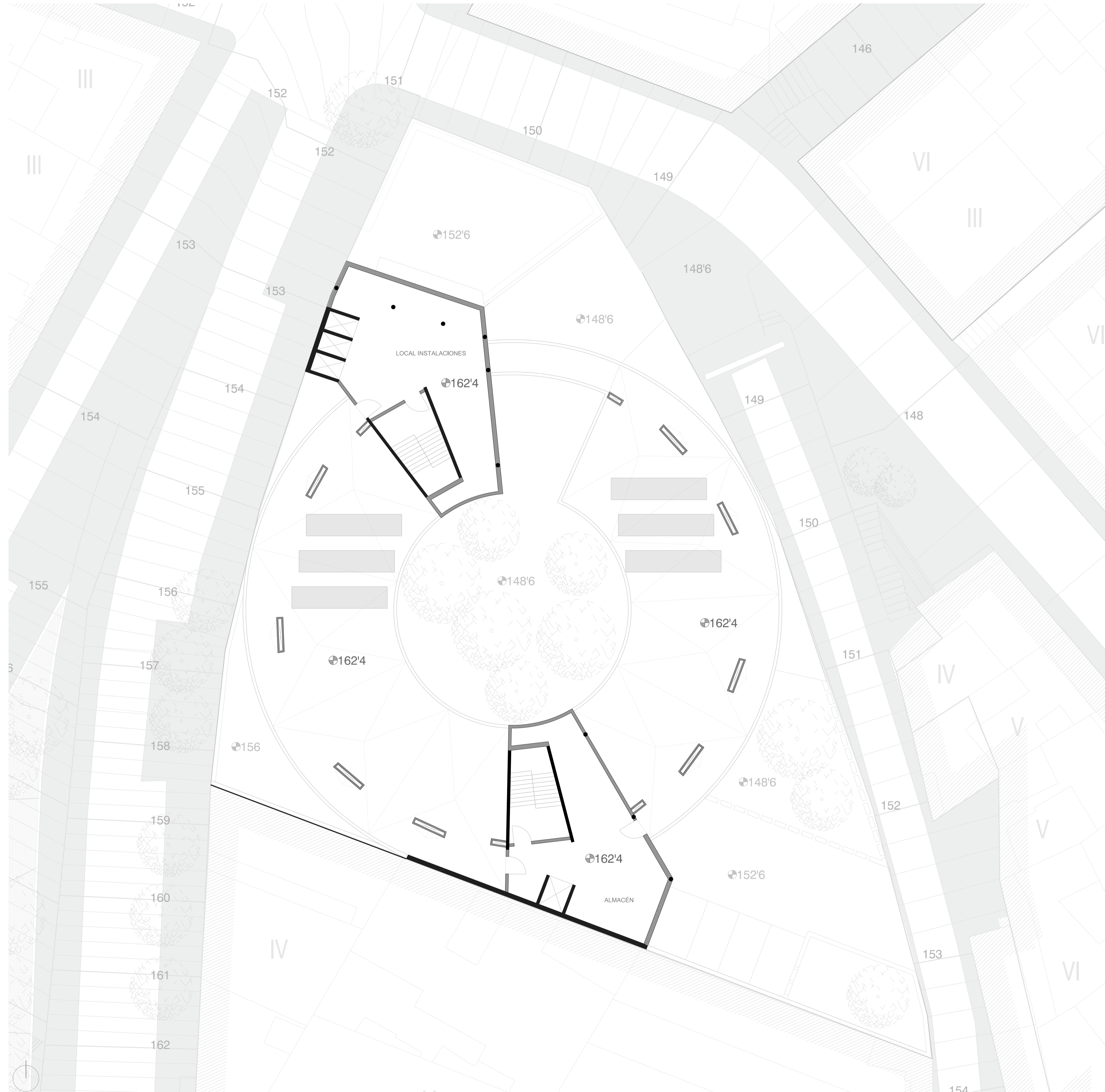
PLANTA CUBIERTA E 1:150
