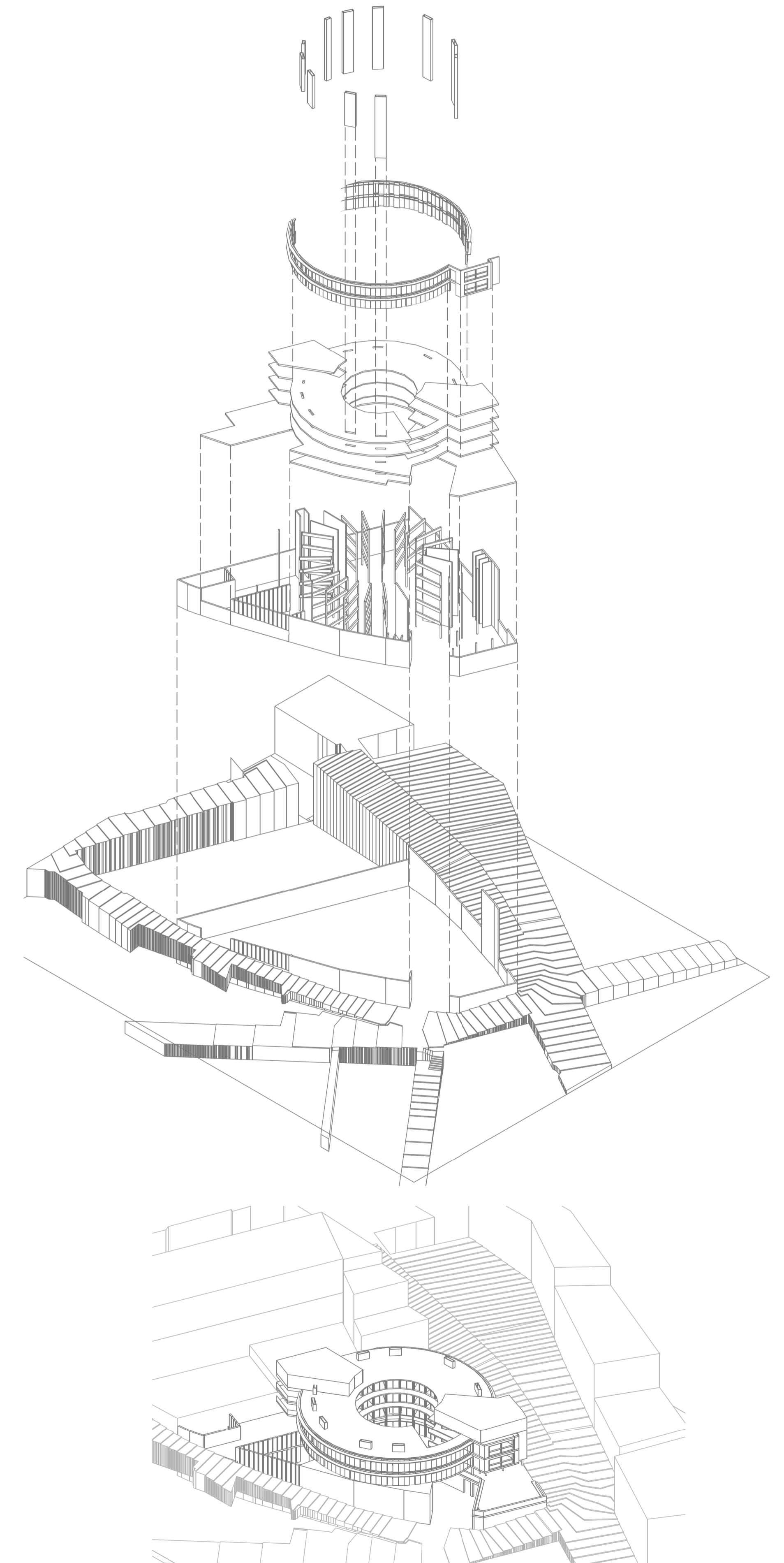
ESQUEMA VOLUMÉTRICO DE LA RELACIÓN ENTRE SISTEMAS TERRENO/ESTRUCTURA VERTICAL/FORJADOS/ENVOLVENTE/INSTALACIONES
