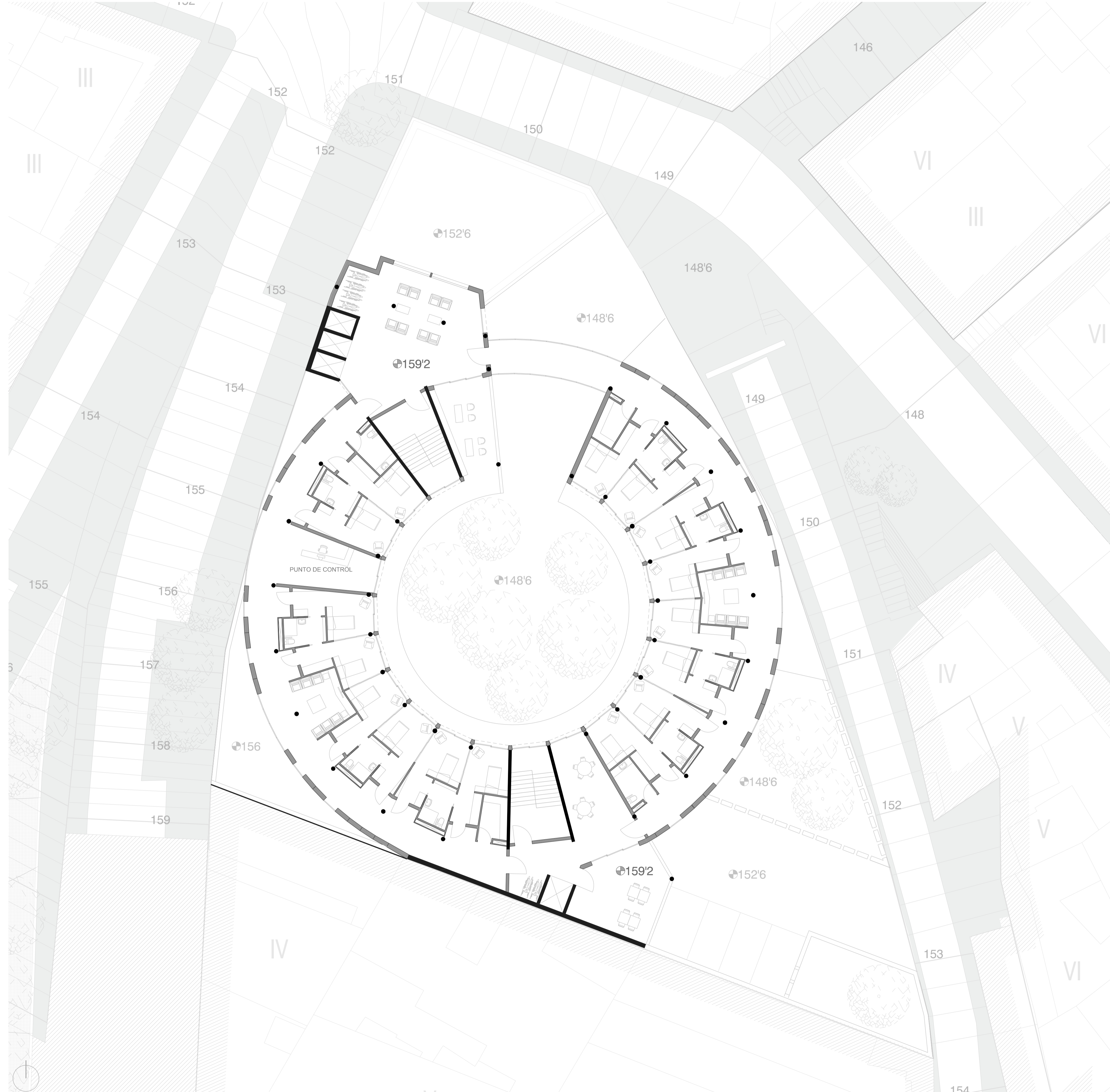
PLANTA TERCERA E 1:150
