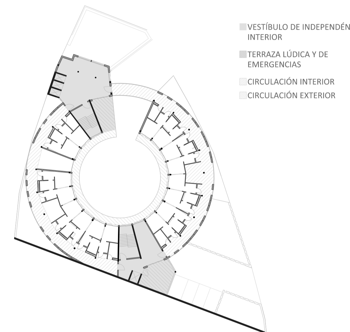
PLANTA CIRCULACIONES Y ACCESOS E 1:450
