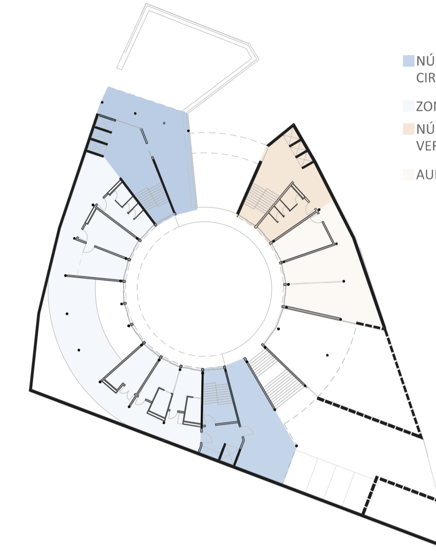
PLANTA USOS E 1:450
