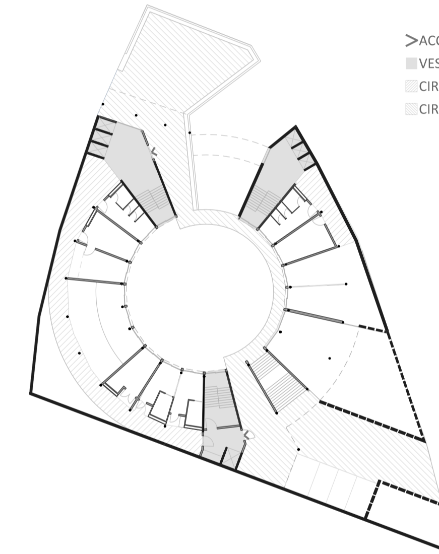
PLANTA CIRCULACIONES Y ACCESOS E 1:450
