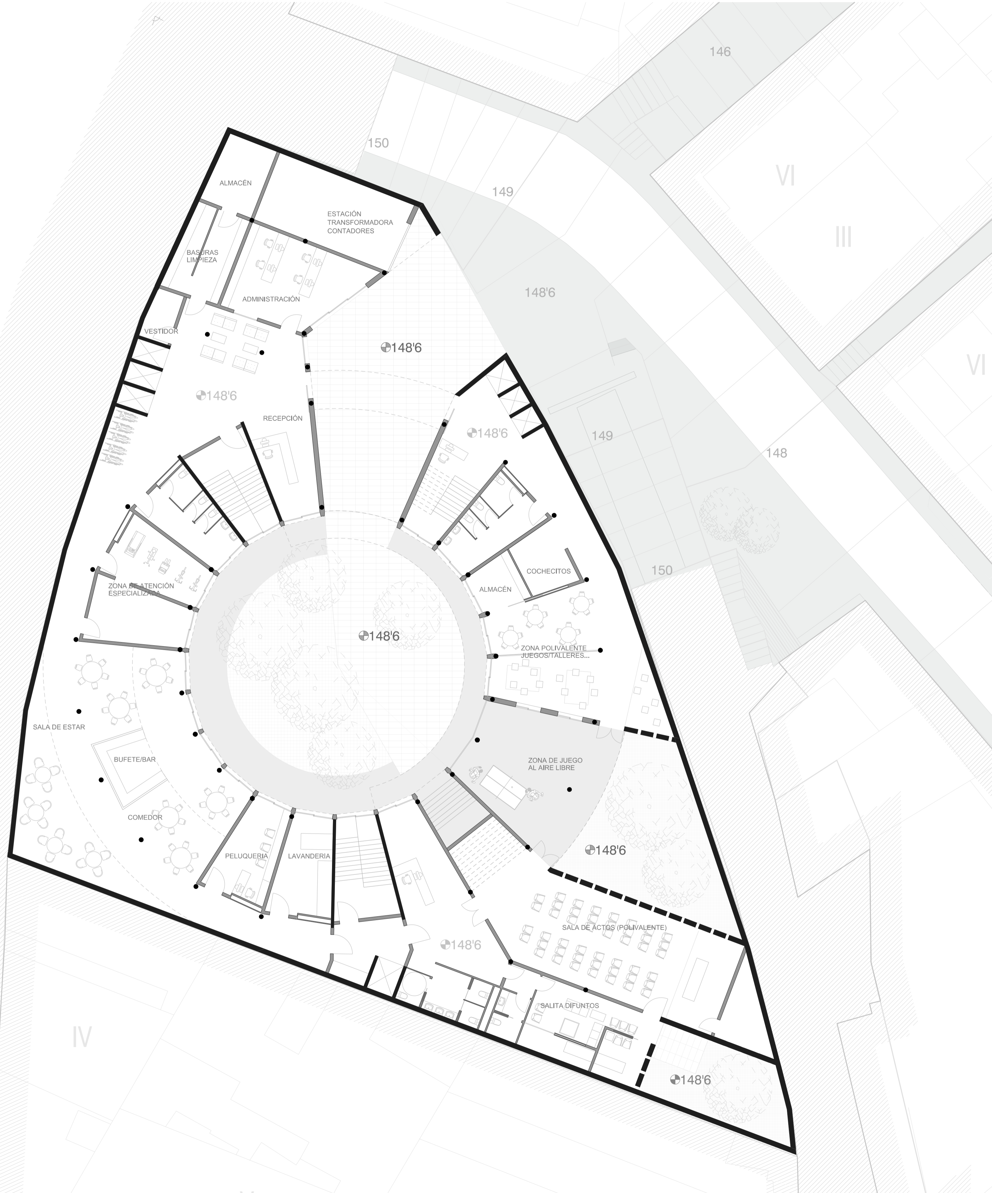
PLANTA CIRCULACIONES Y ACCESOS E 1:450
