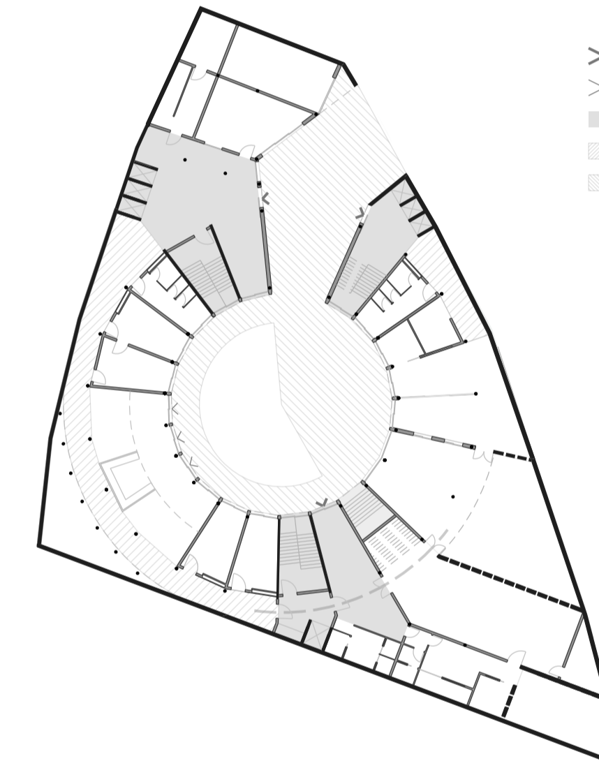
PLANTA CIRCULACIONES Y ACCESOS E 1:450
