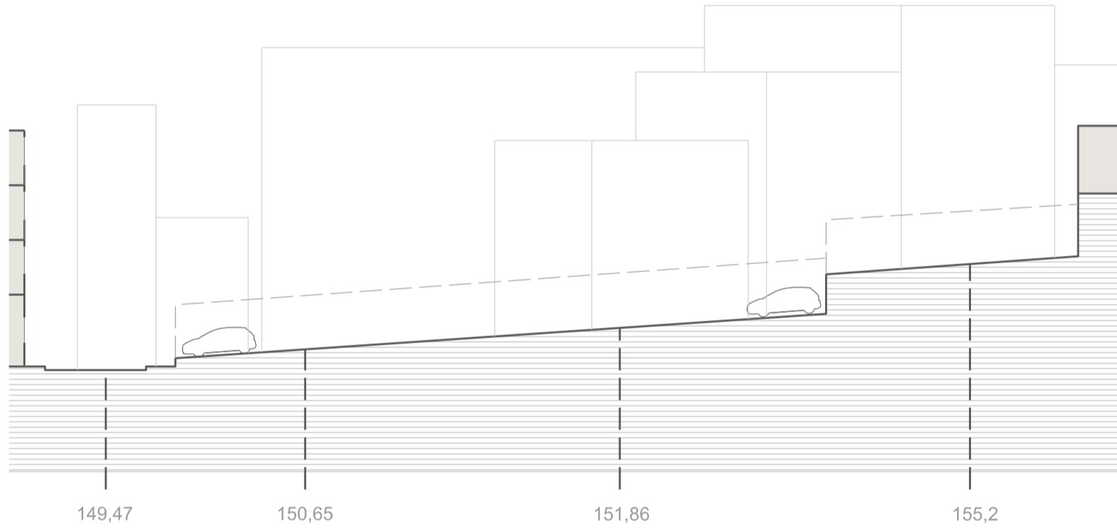
SECCIÓN SOLAR S1-S1' E 1:300
