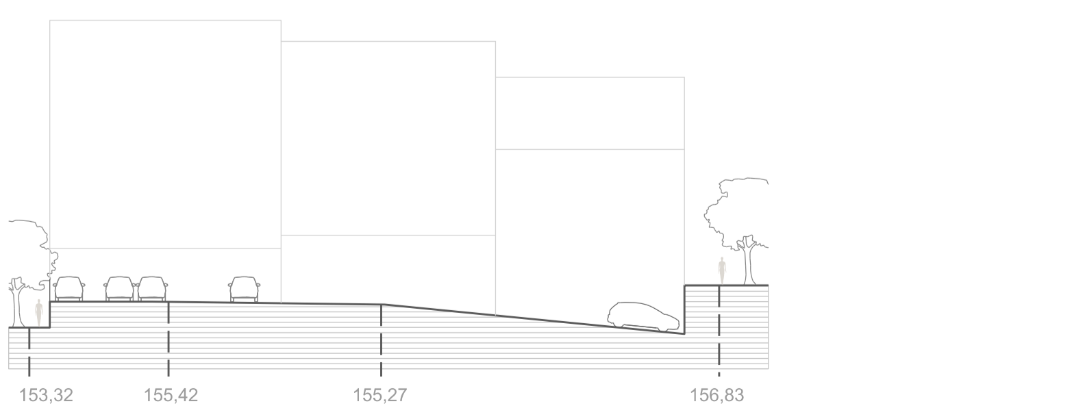
SECCIÓN SOLAR S3-S3' E 1:300
