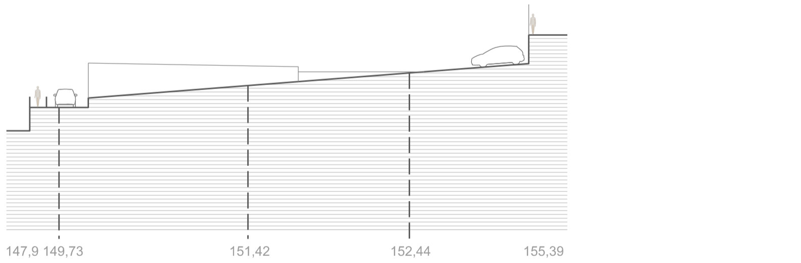
SECCIÓN SOLAR S2-S2' E 1:300
