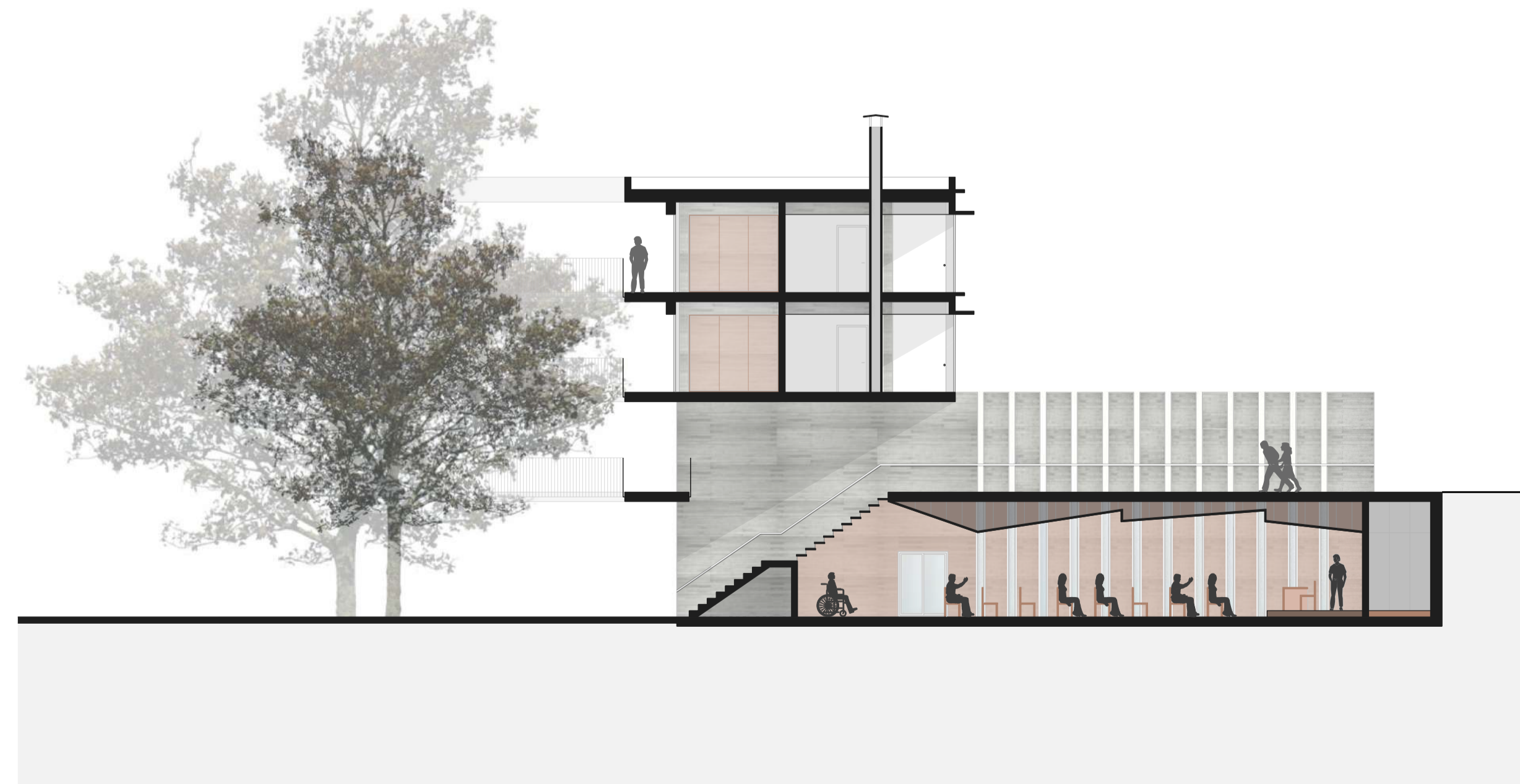
SECCIÓN S2-S2'. SALA DE ACTOS/ESCALERA E 1:150
