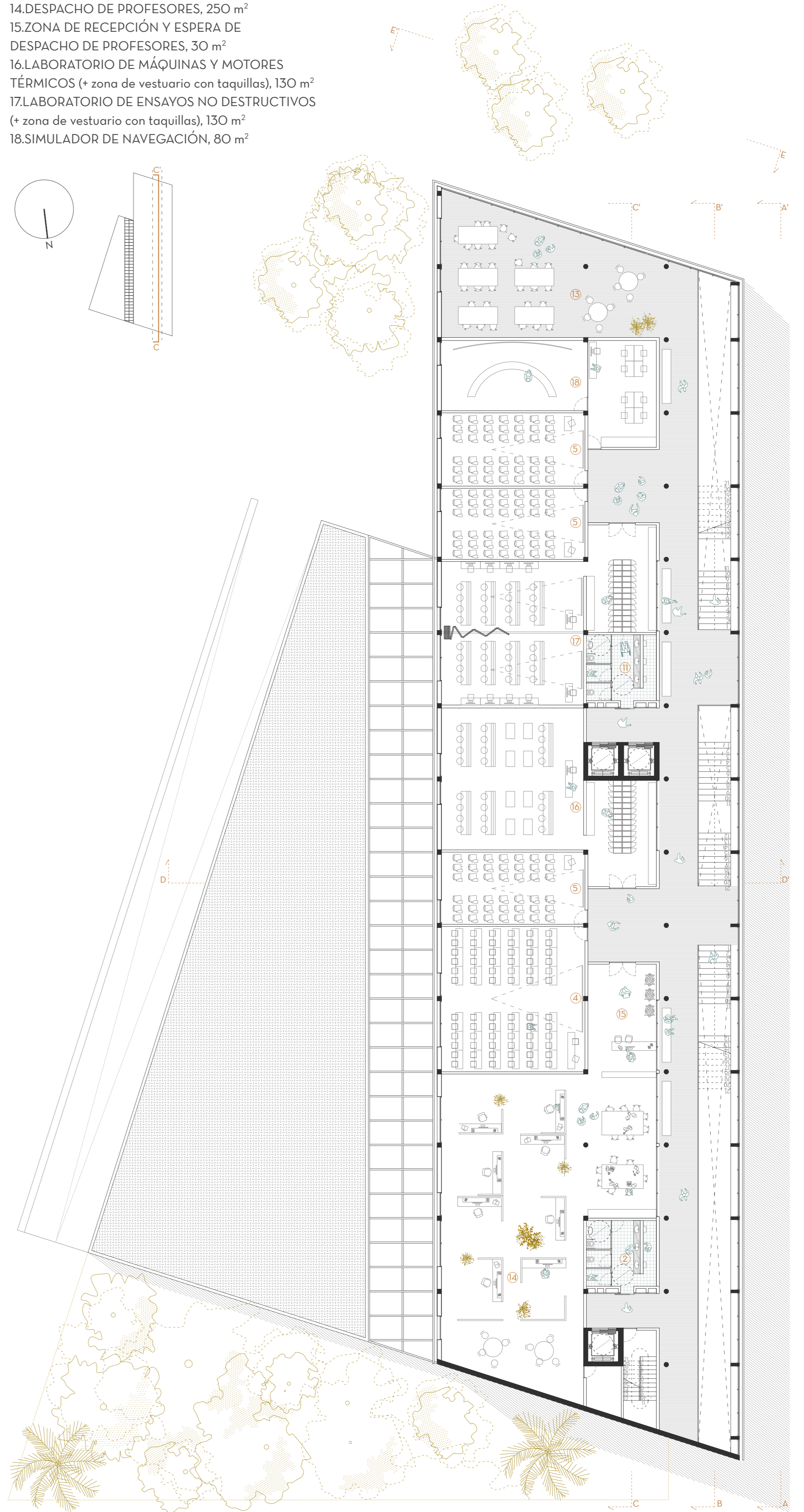
planta tercera (+13,50)
