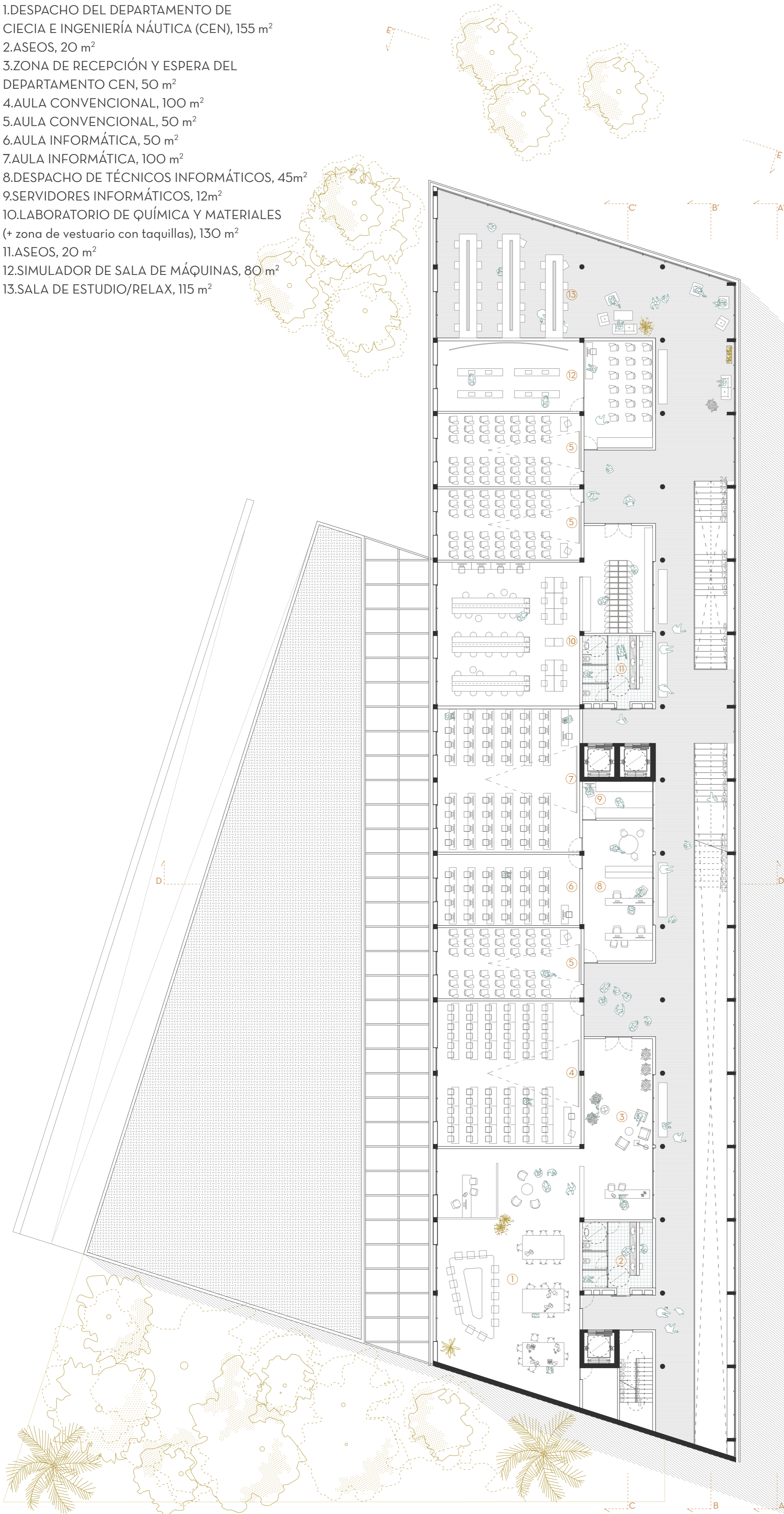
planta segunda (+10,00)
