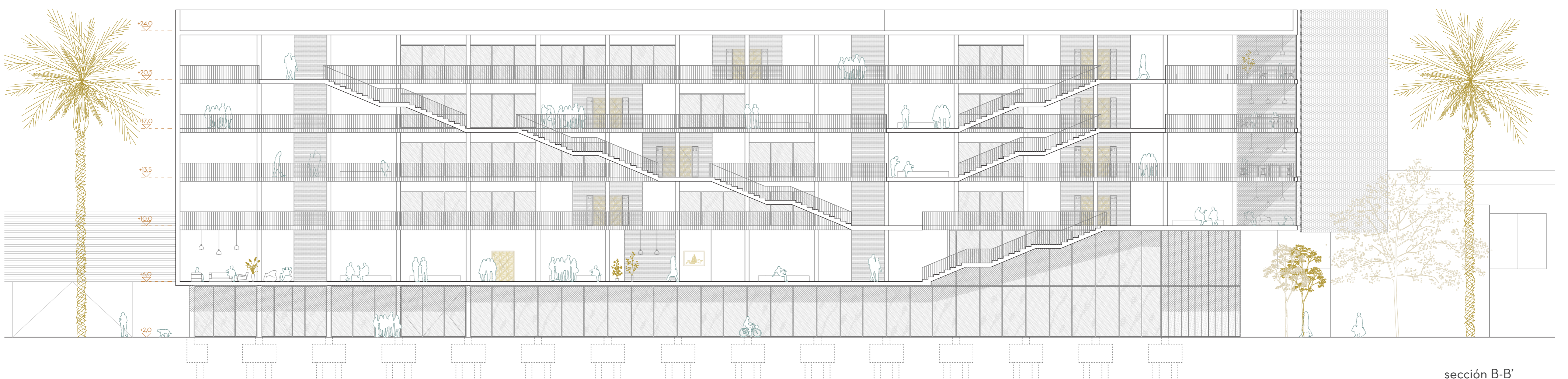
sección B-B'
