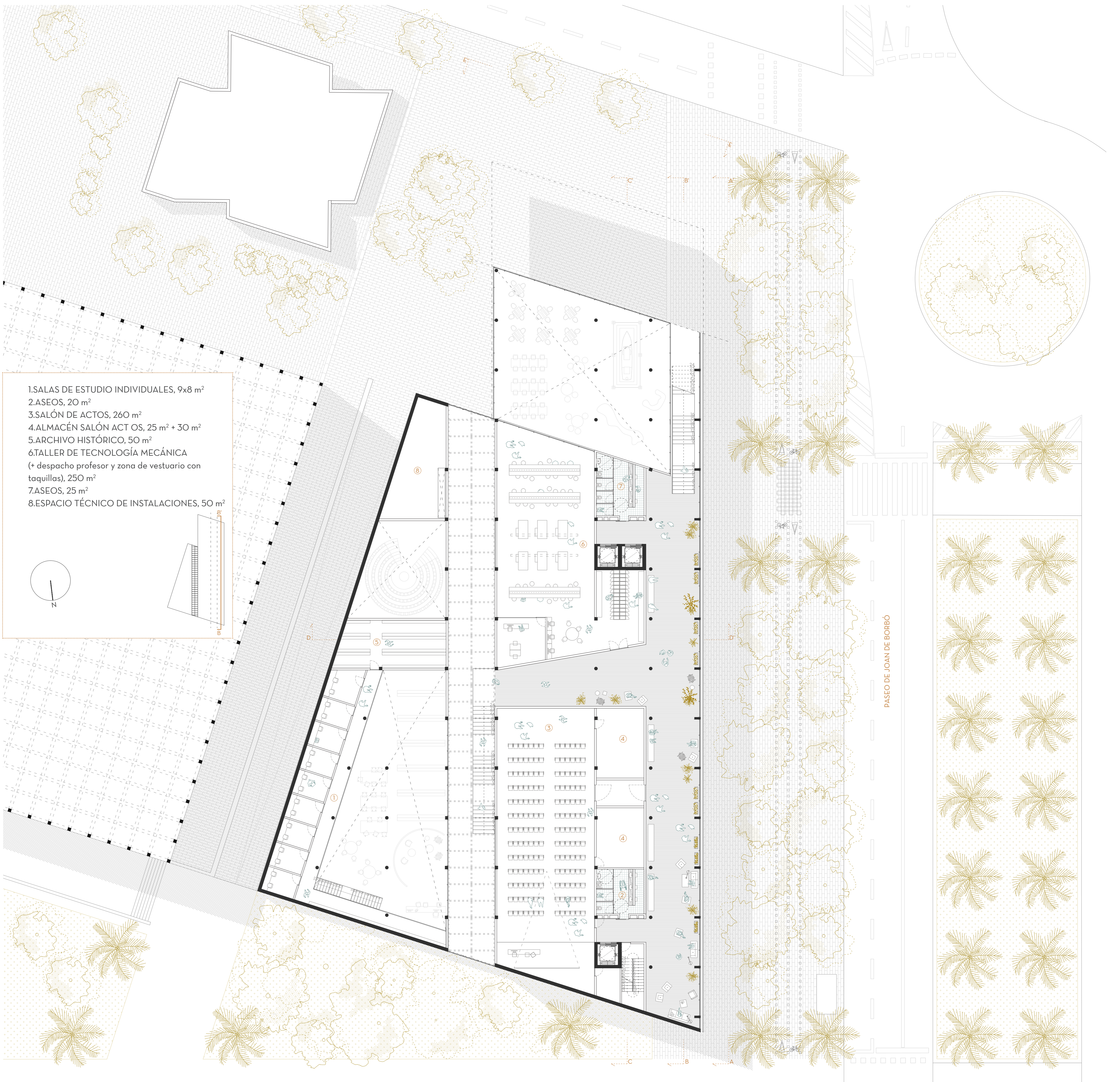
planta primera (+6,00)
