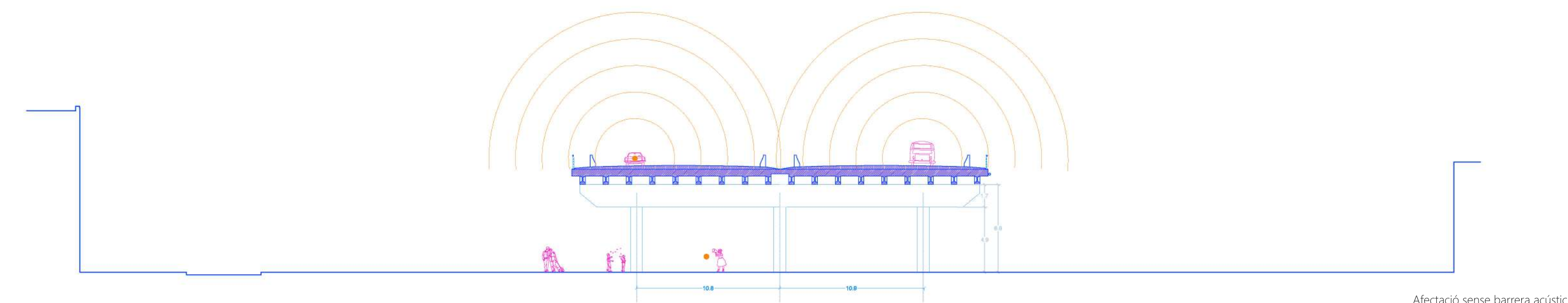
Afectació sense barrera acústica
