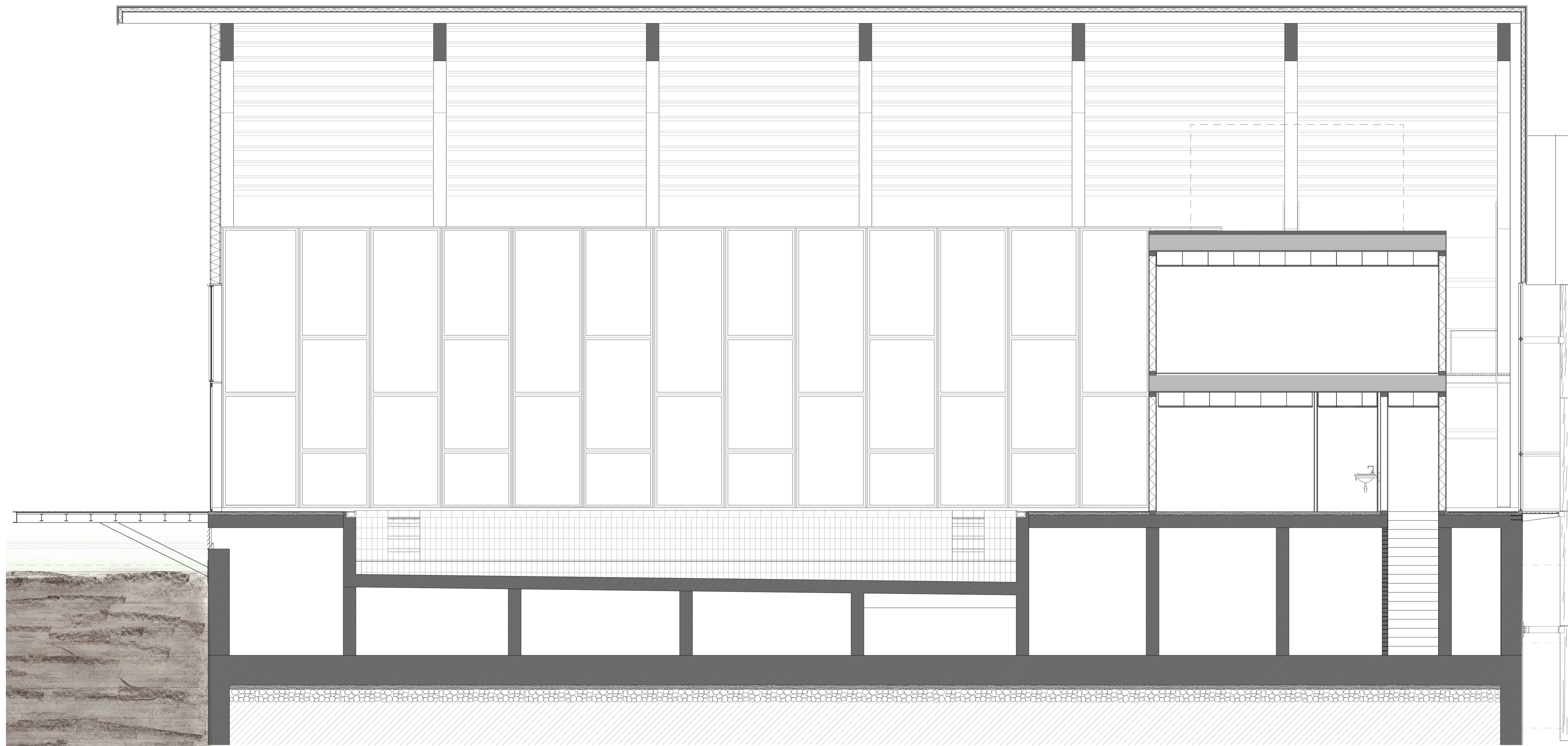
SECCION A-A'
