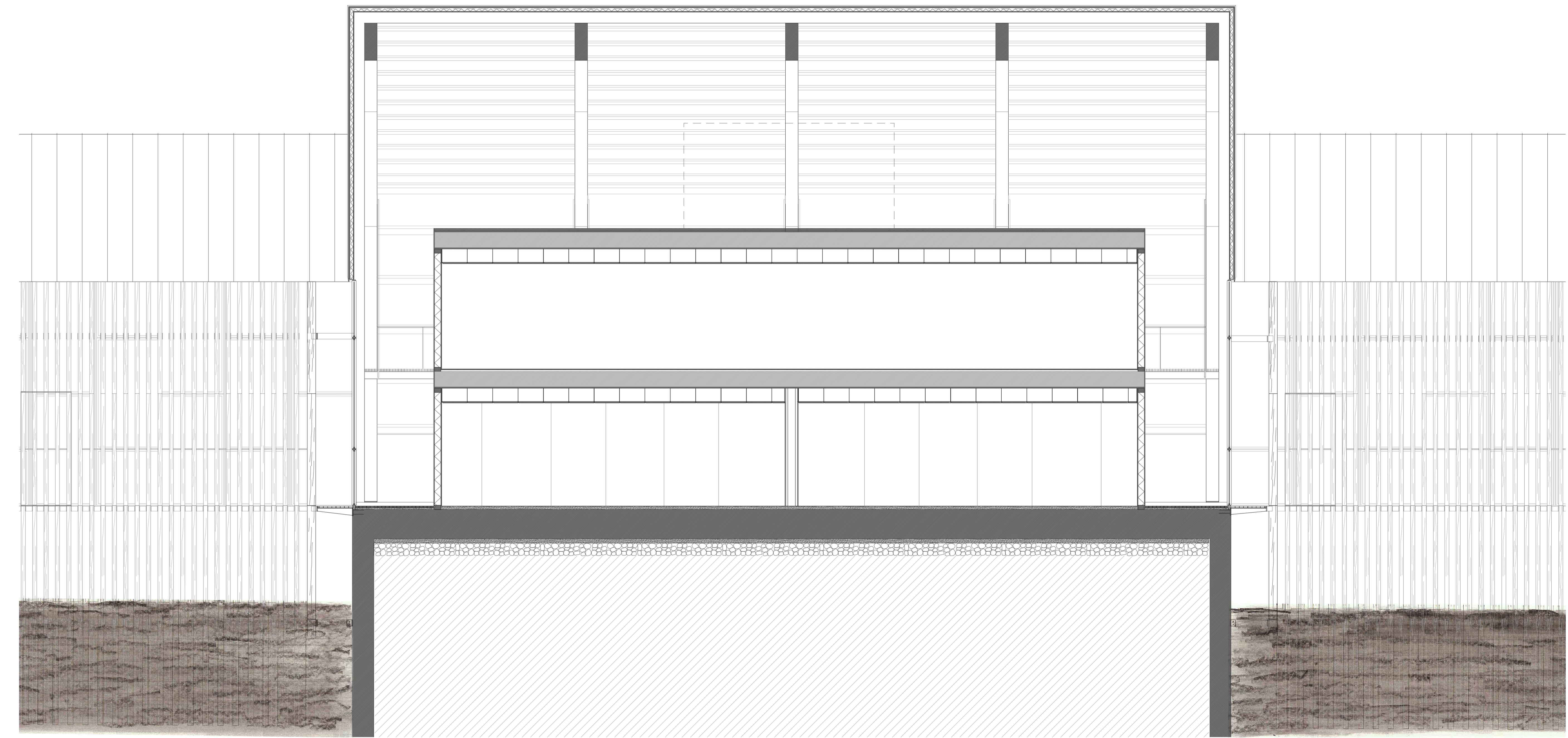
SECCION B-B'
