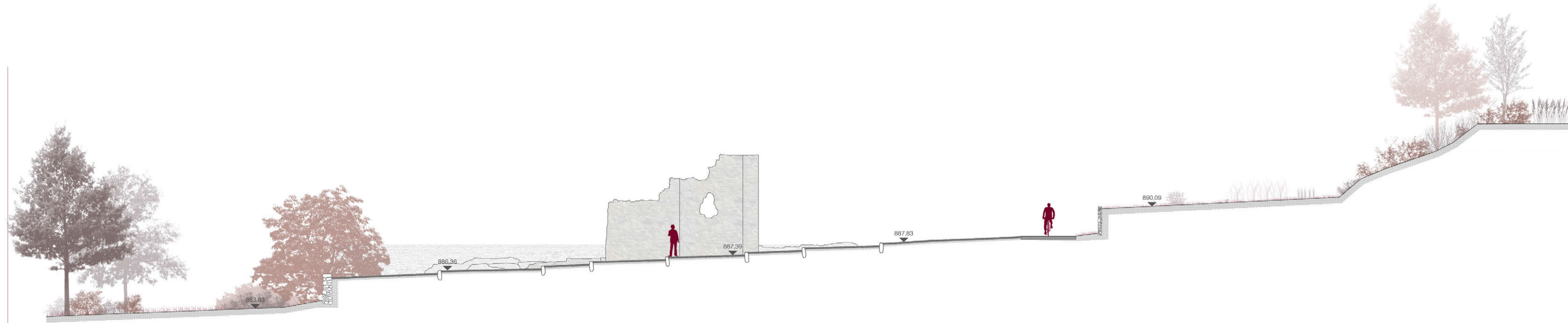
SECCIÓ AA' E: 1/100
