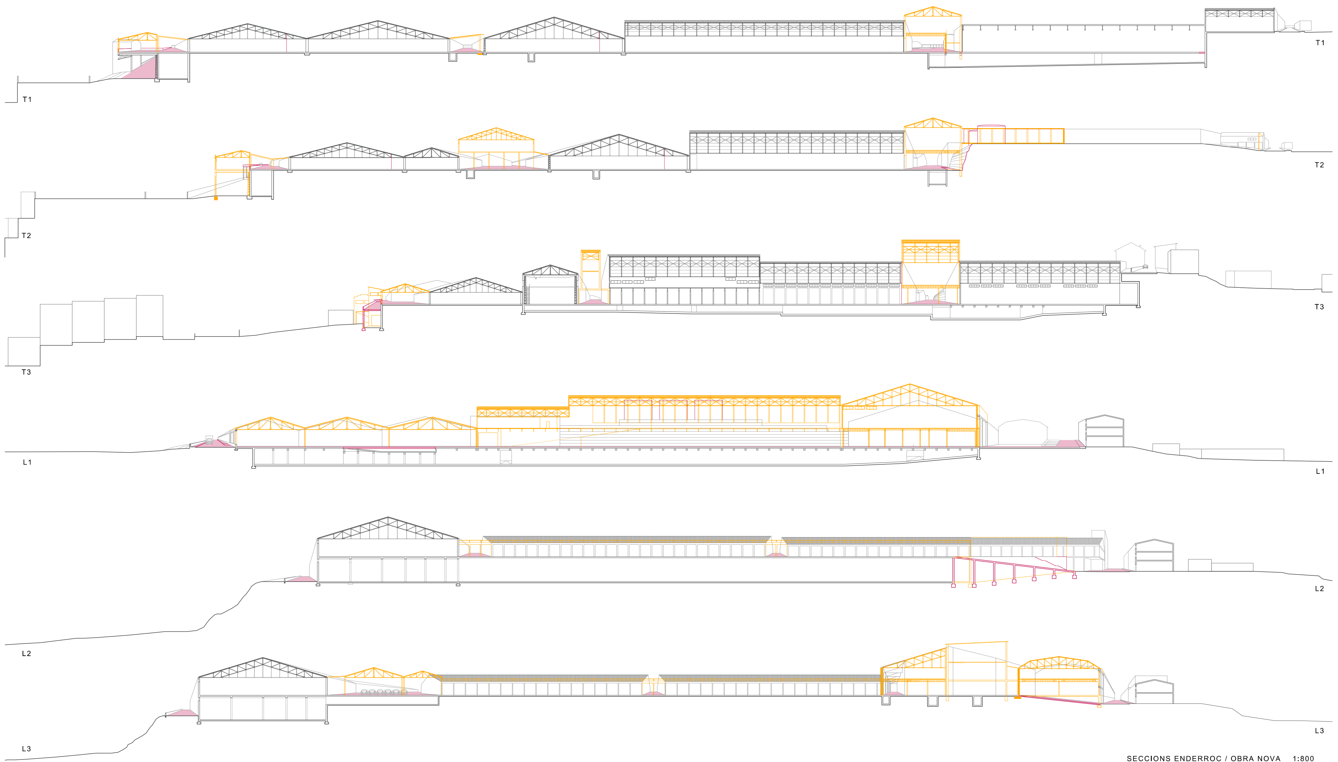
SECCIONS ENDERROC / OBRA NOVA 1:800
