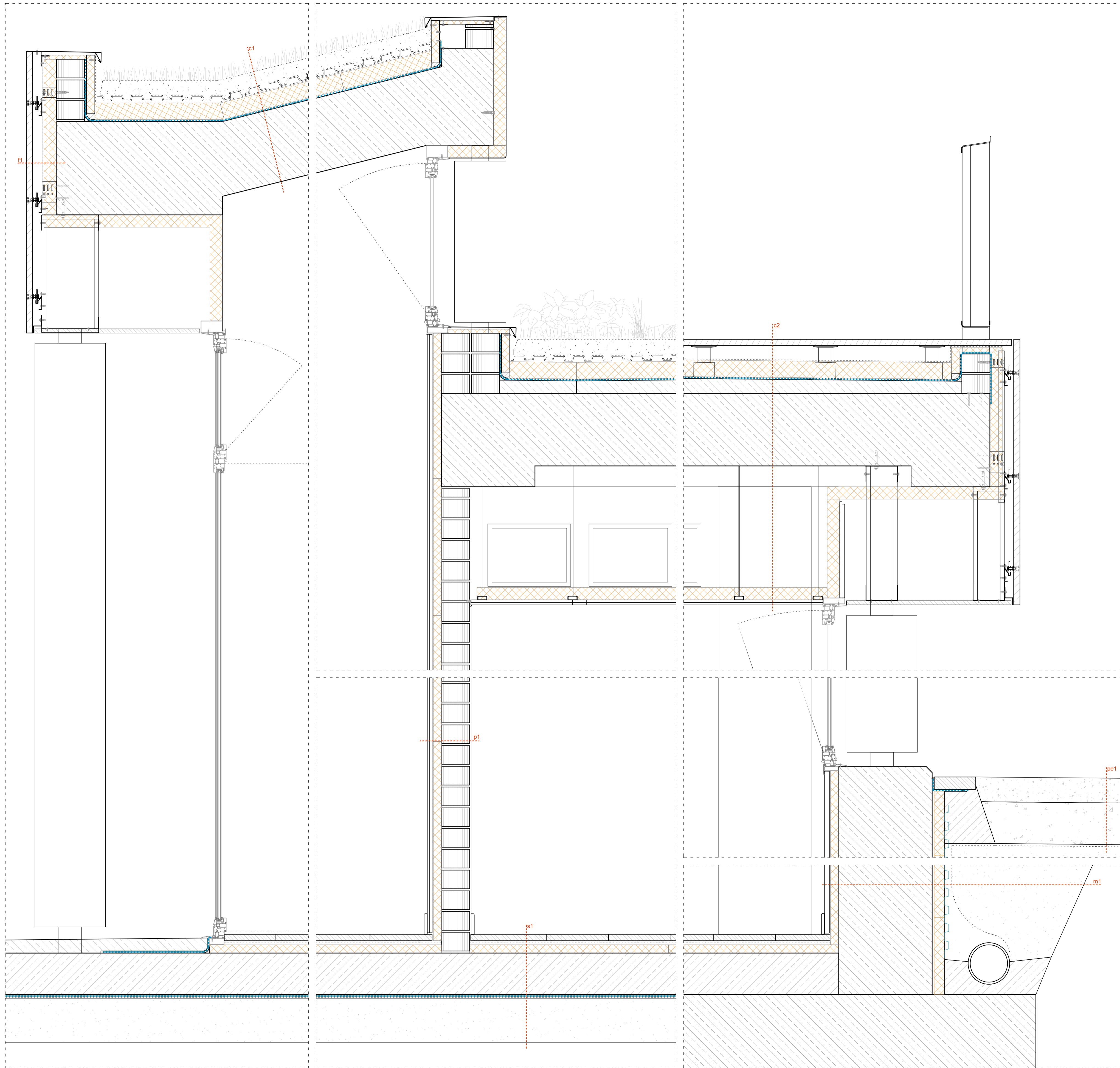
SECCIÓN TALLER Y LUDOTECA
