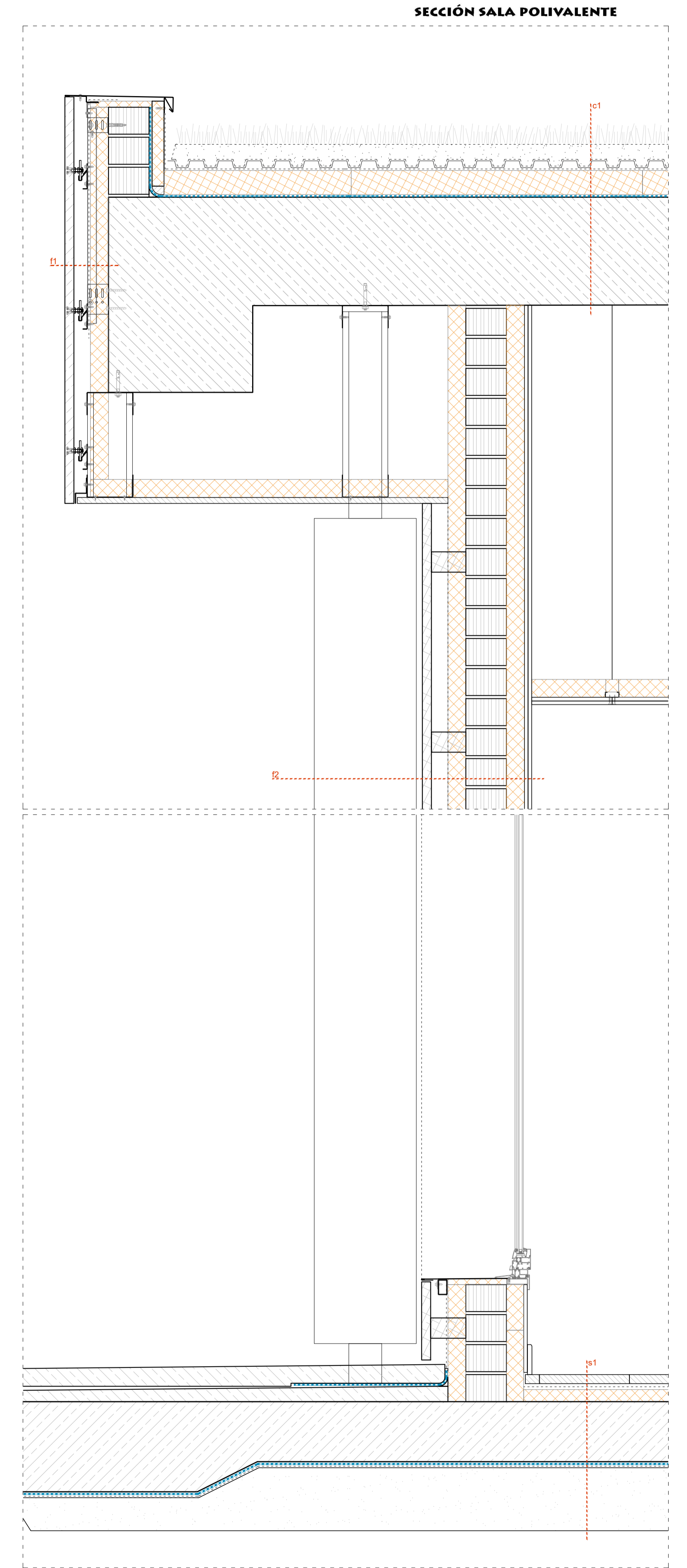
SECCIÓN SALA POLIVALENTE
