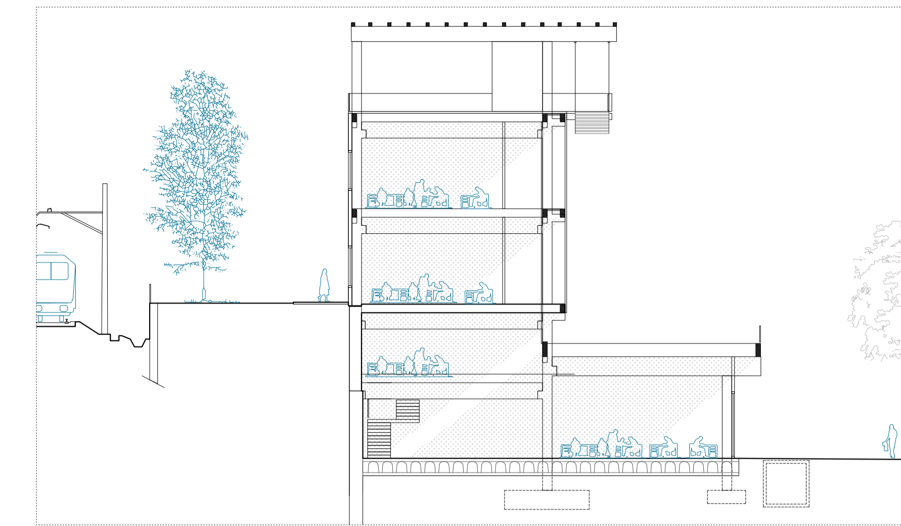
Sección tipo 4
