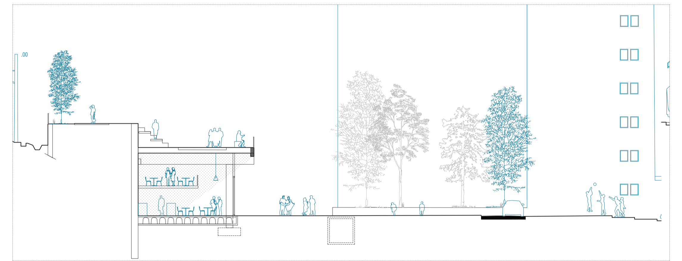
Sección tipo 3
