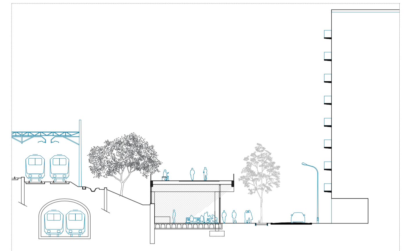
Sección tipo 1
