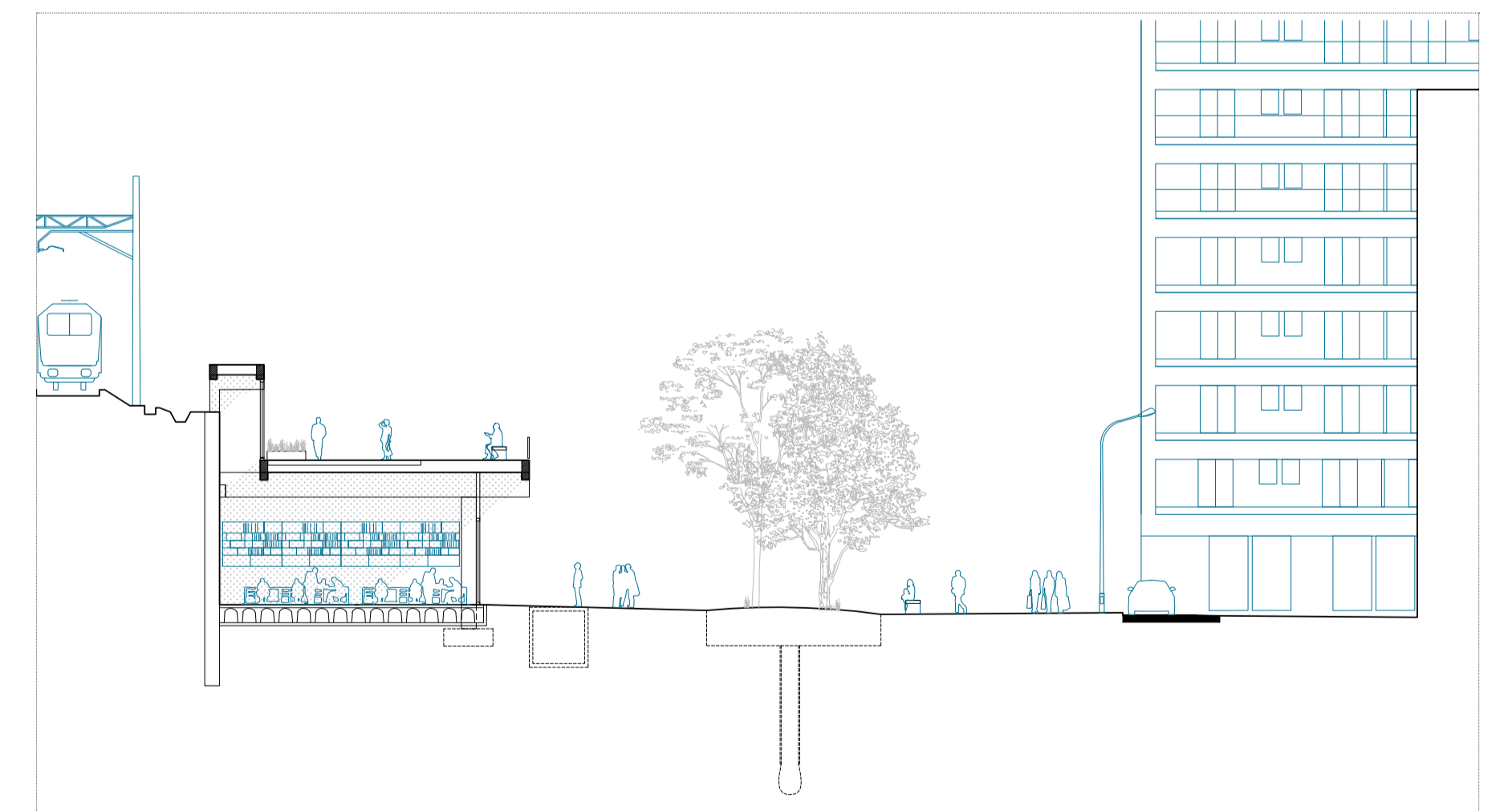
Sección tipo 2
