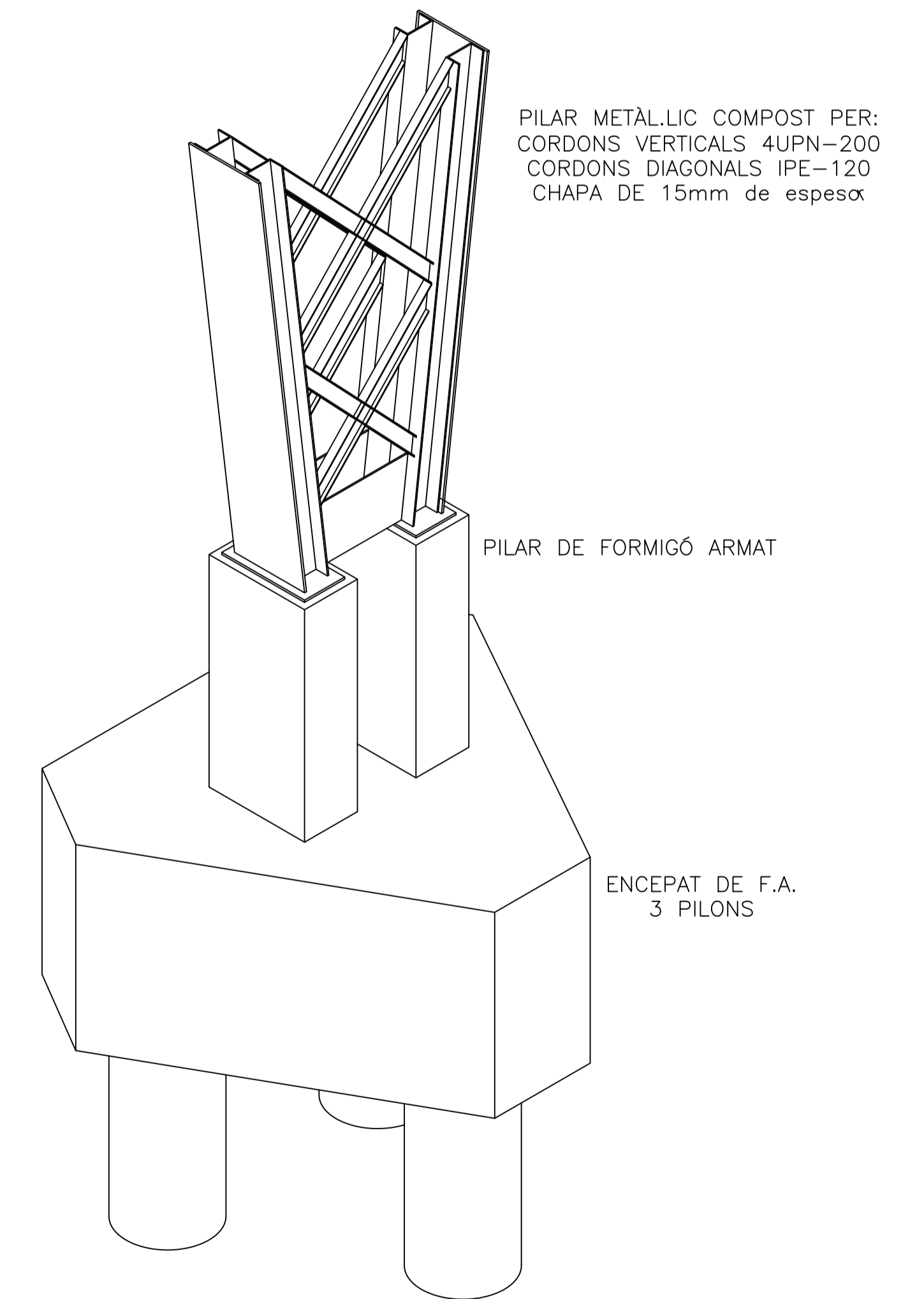
ESQUEMA PILAR PLANTA BAIXA EDIFICI PRINCIPAL
