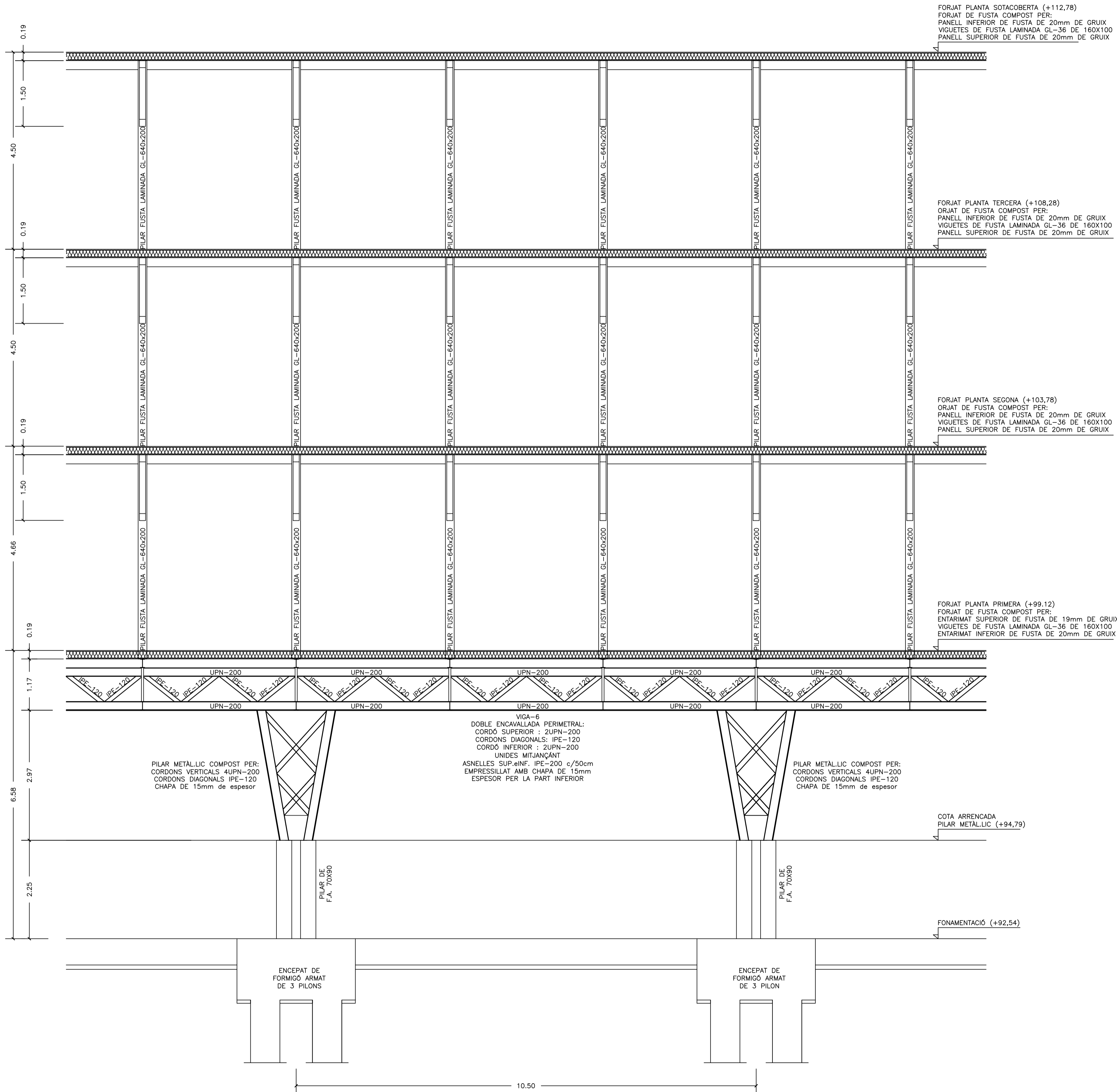
ESQUEMA PILAR PLANTA BAIXA EDIFICI PRINCIPAL
