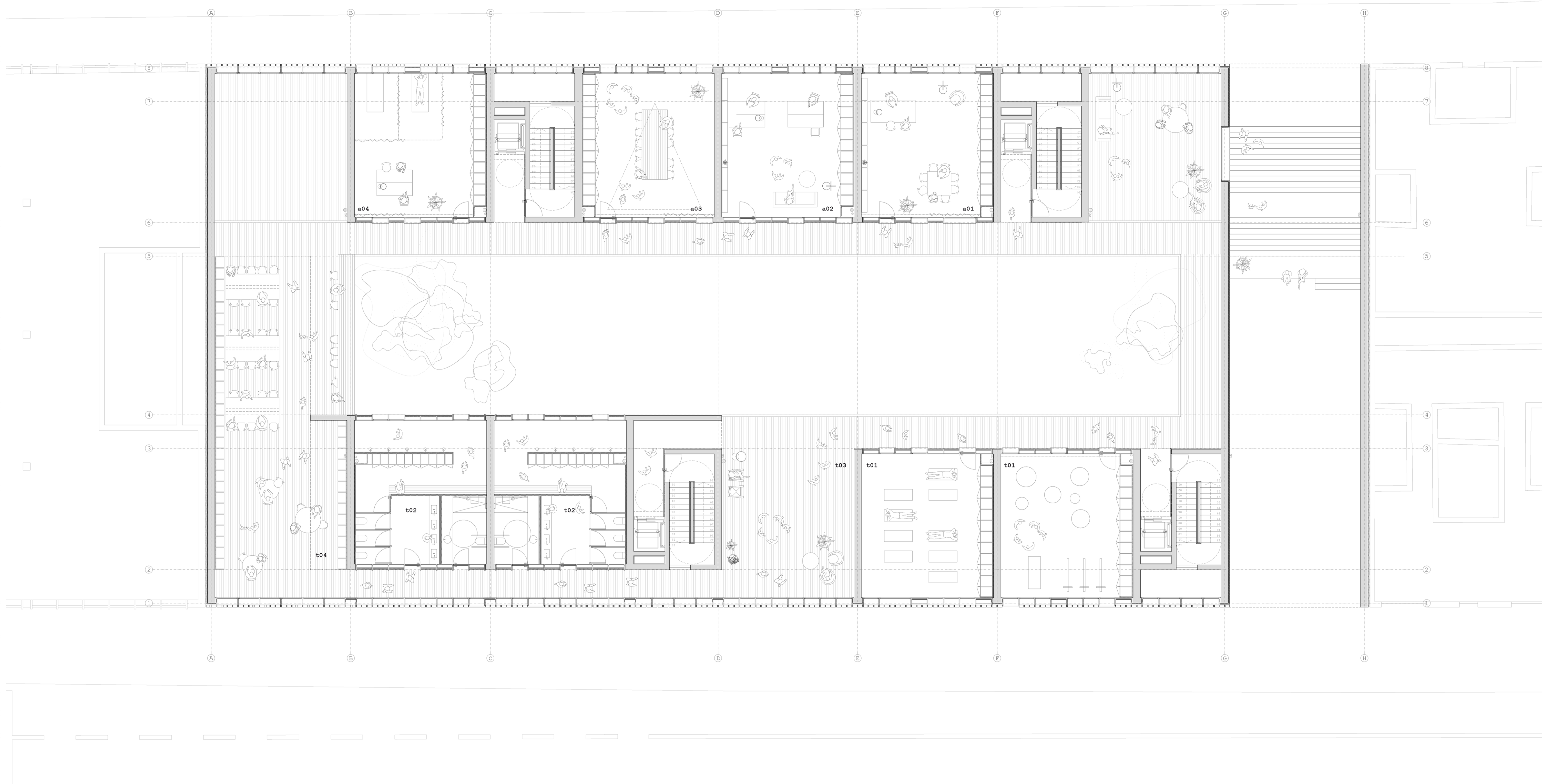
planta primera 1:100
