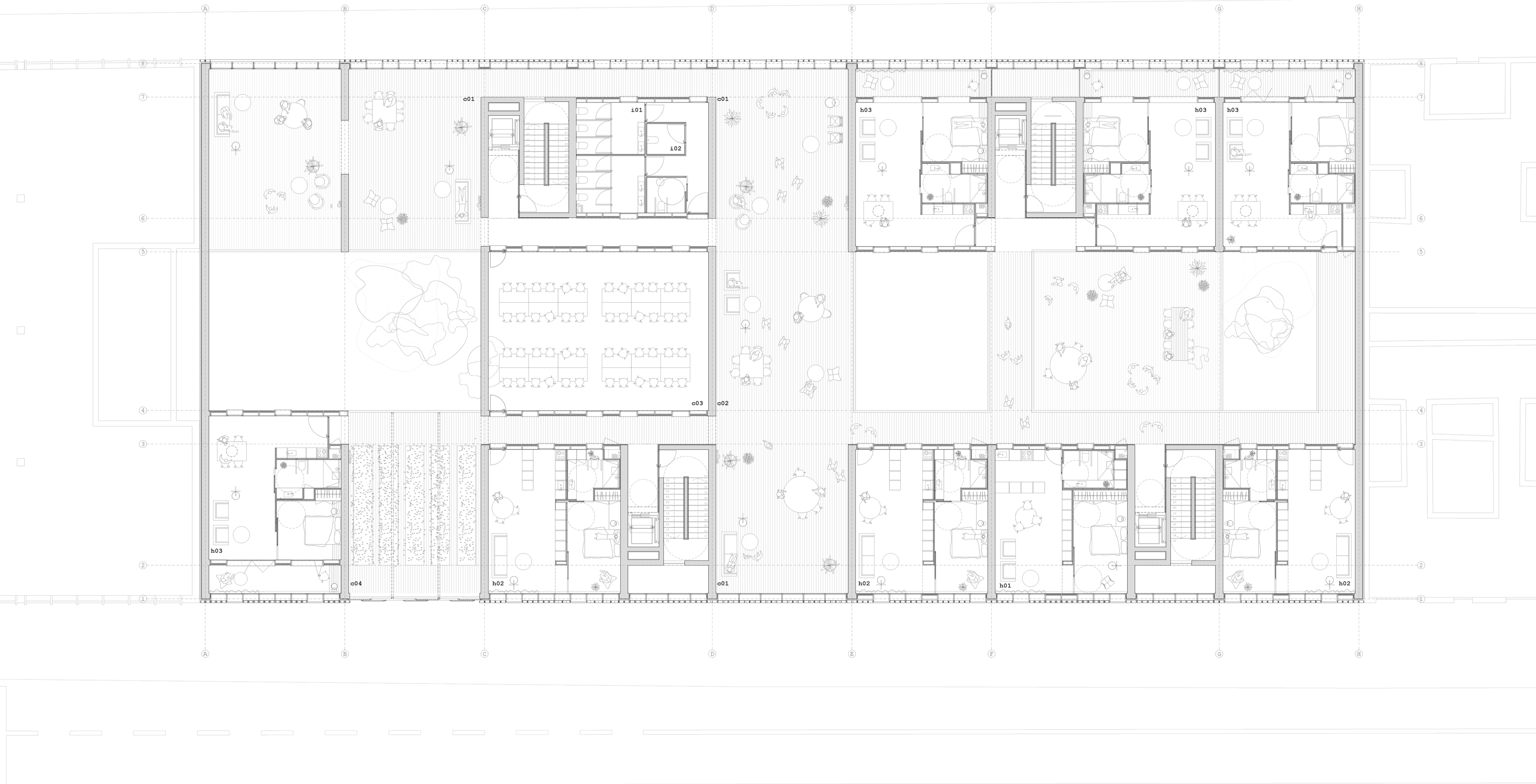
planta cinquena 1:100
