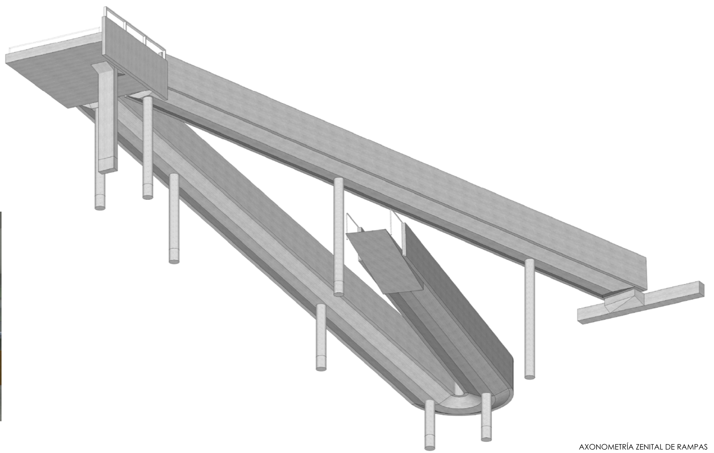
AXONOMETRÍA ZENITAL DE RAMPAS
