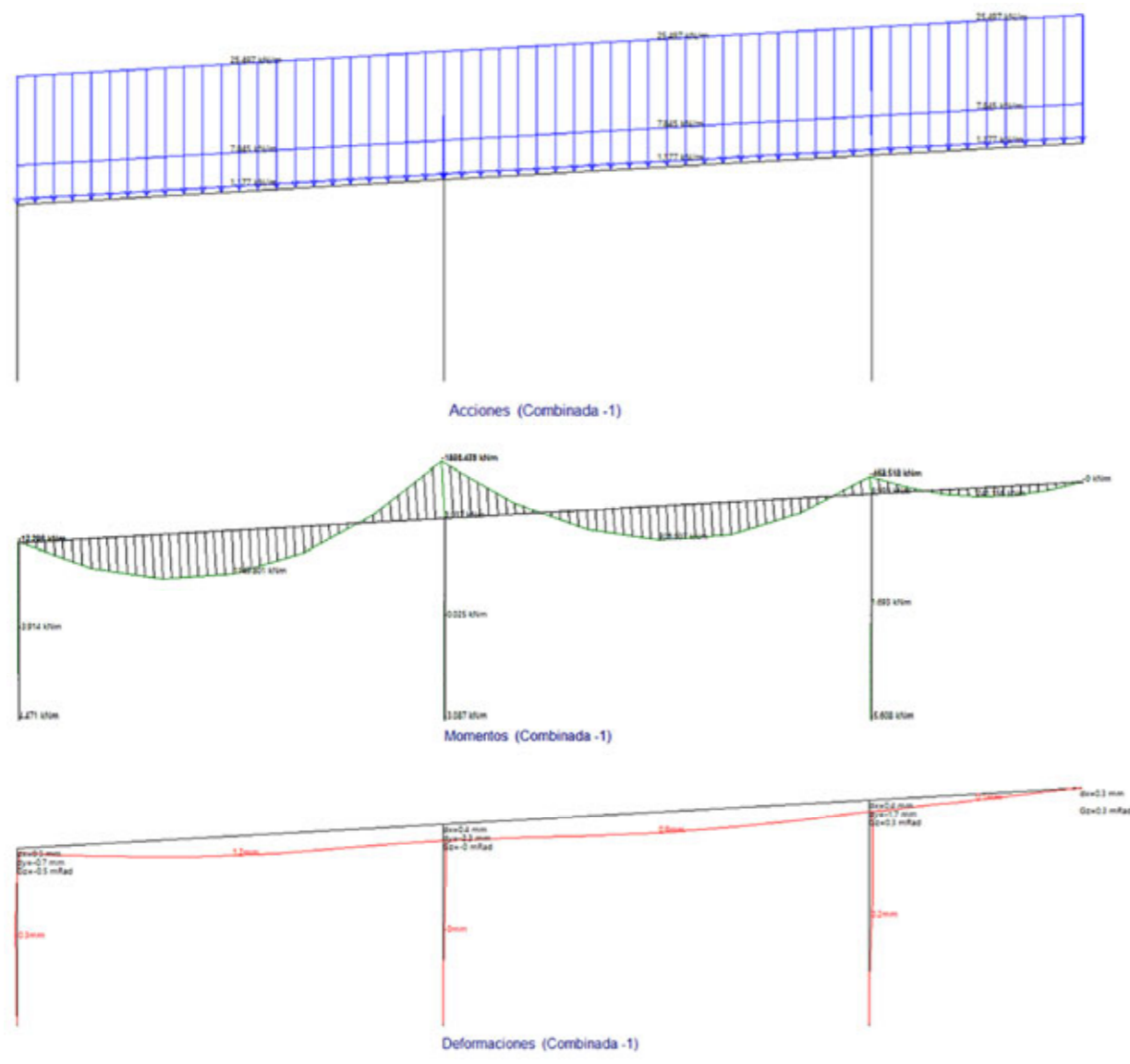
ESQUEMAS ESTRUCTURALES DE CÁLCULO TRAMO SUPERIOR DE RAMPA
