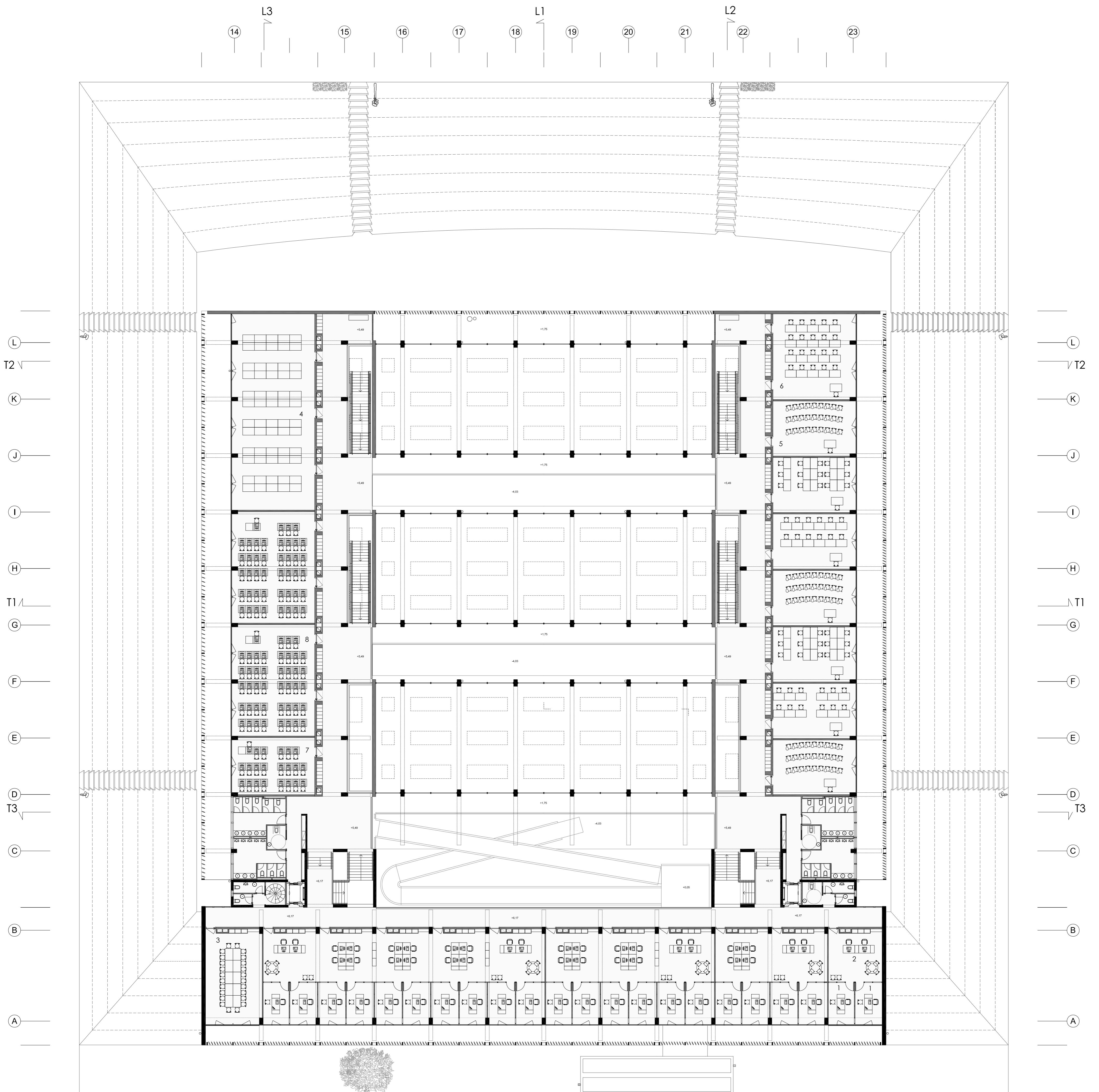
PLANTA cotas +5.49 y 6.17 m Niveles Aulas 2 y Departamentos 3
