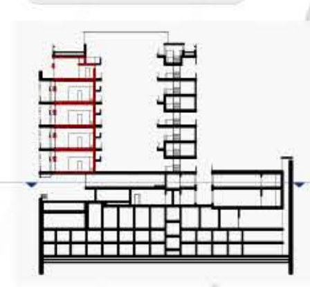
planta entressòl
