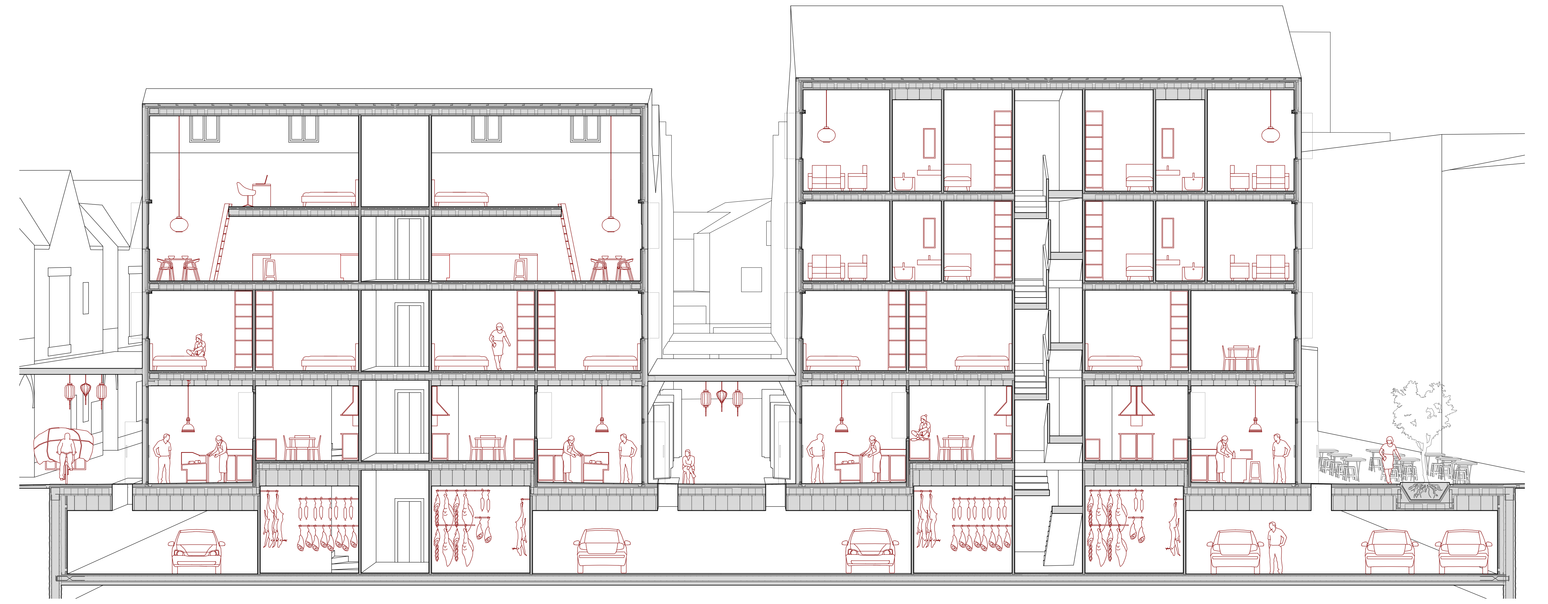
Secció E 1/75
