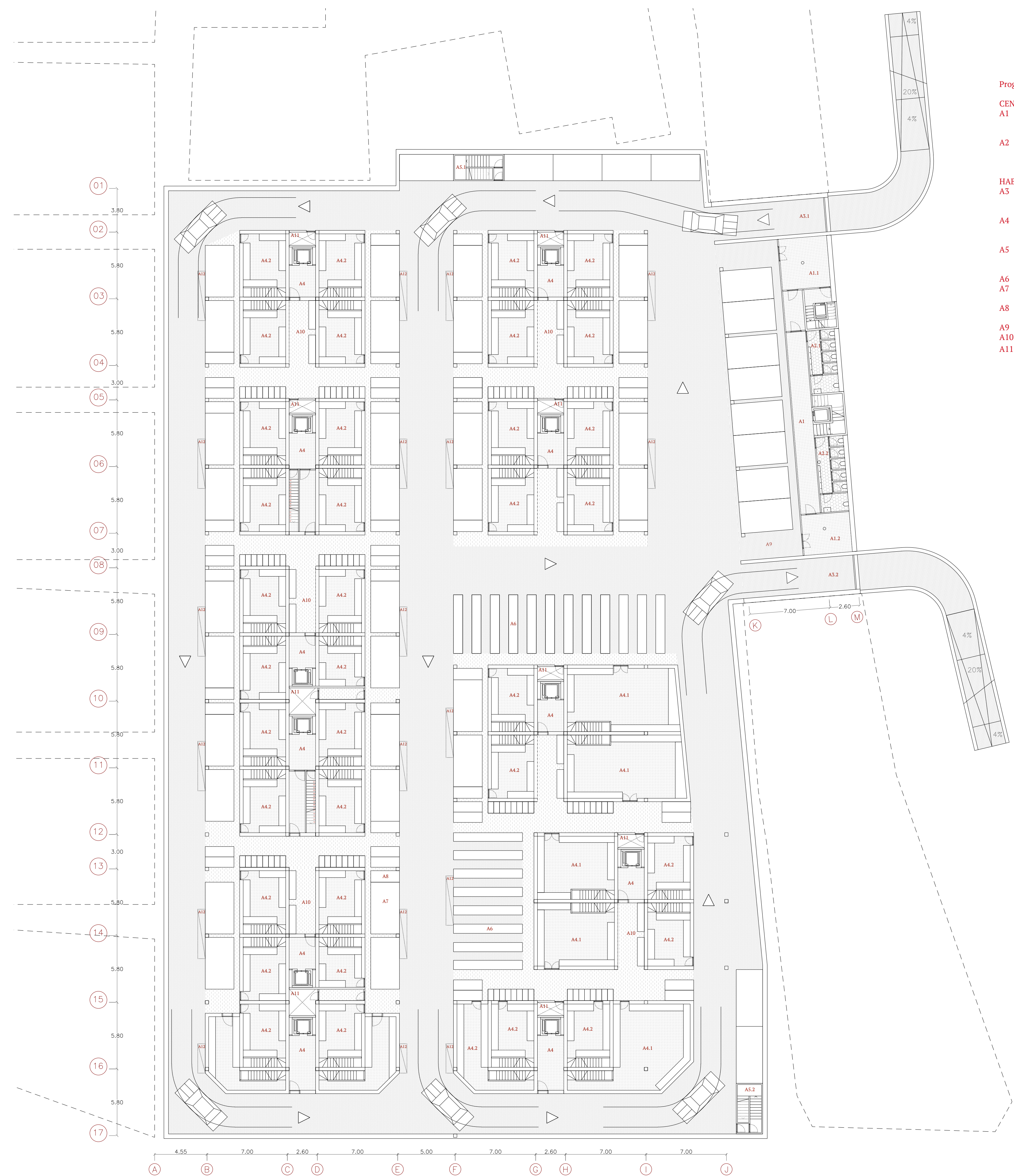
Planta Soterrani -5m E 1/200
