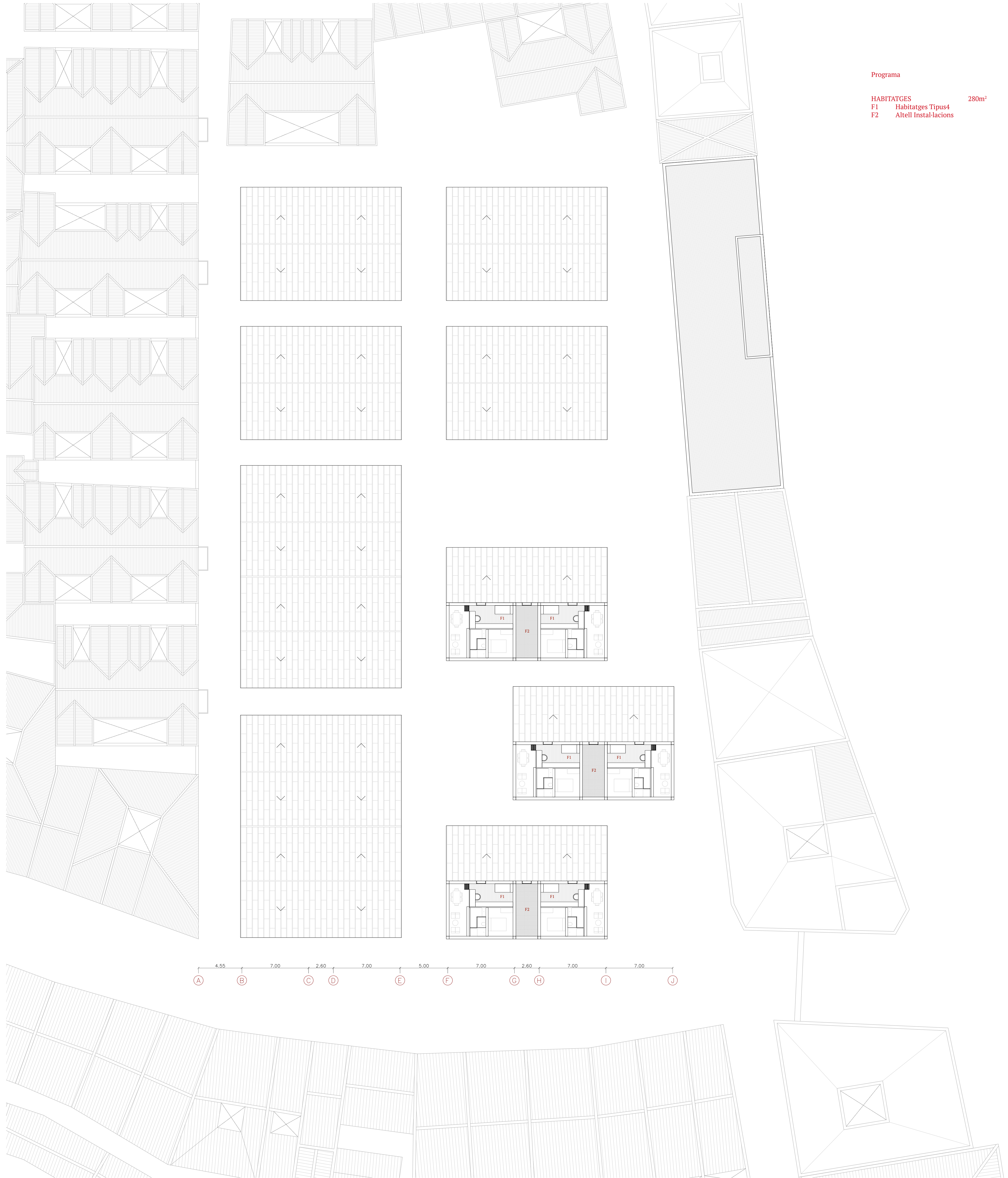
Planta Atells +12m E 1/200
