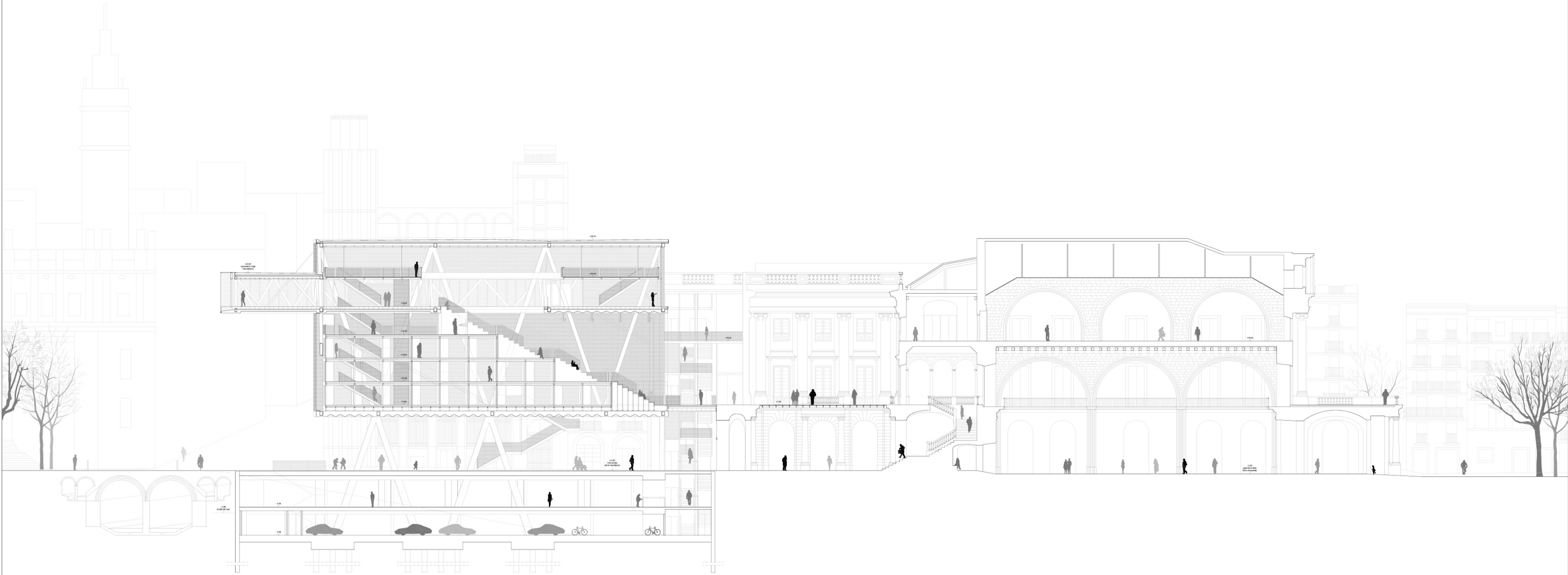
1. Secció Longitudinal E1.150.
