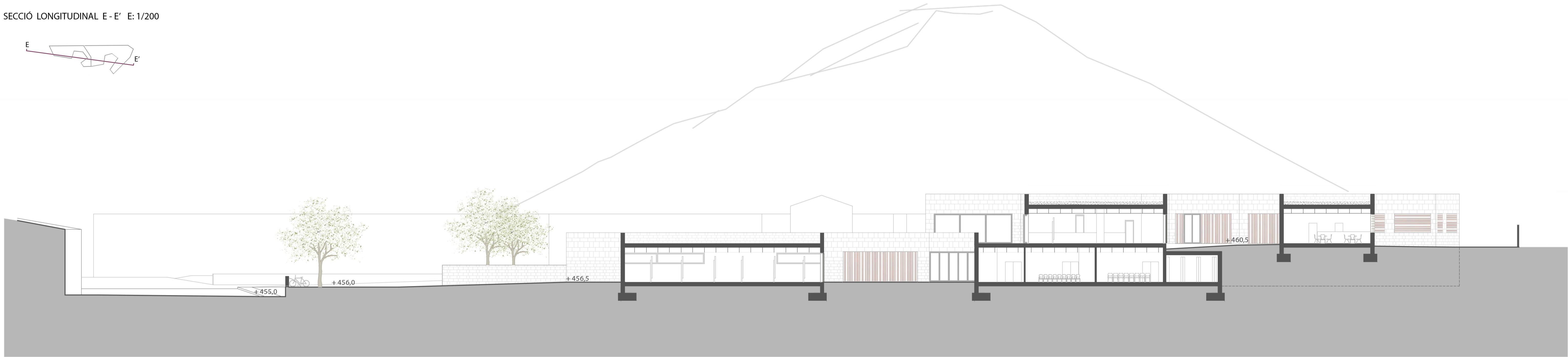
SECCIÓ LONGITUDINAL F - F' E: 1/200
