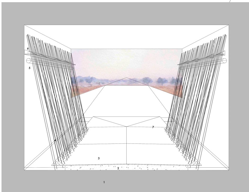
1. Estructura túnel exterior. 2. Formigó de pendent. 3. Placa d'acer perforada en els extrems. 4 Rodons d'acer. 5. sistema il·luminació 6. suport superior prefabricat d'acer. 7. Placa d'adaptació al pendent
