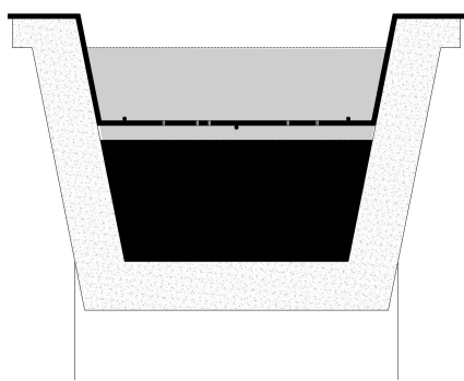
Detall de la passarel·la de vianants en acer E 1:30
