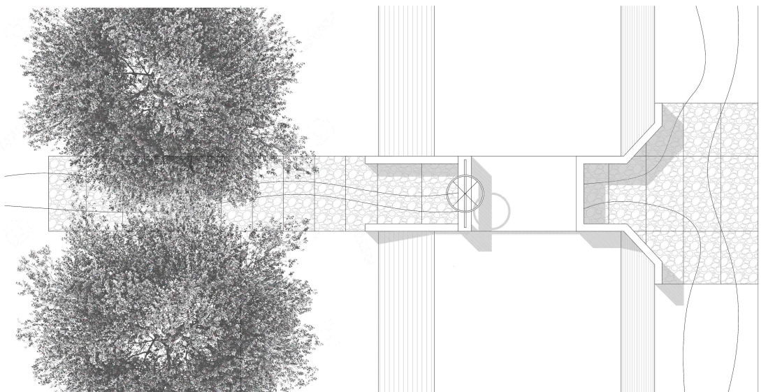
Planta de la comporta i canal de drenatge
